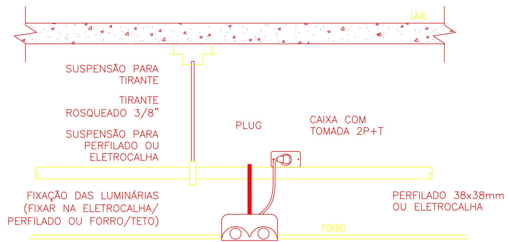
LIGAÇÃO DAS LUMINÁRIAS EM PERFILADO OU ELETROCALHA SEM ESCALA (dimensões indicadas)
