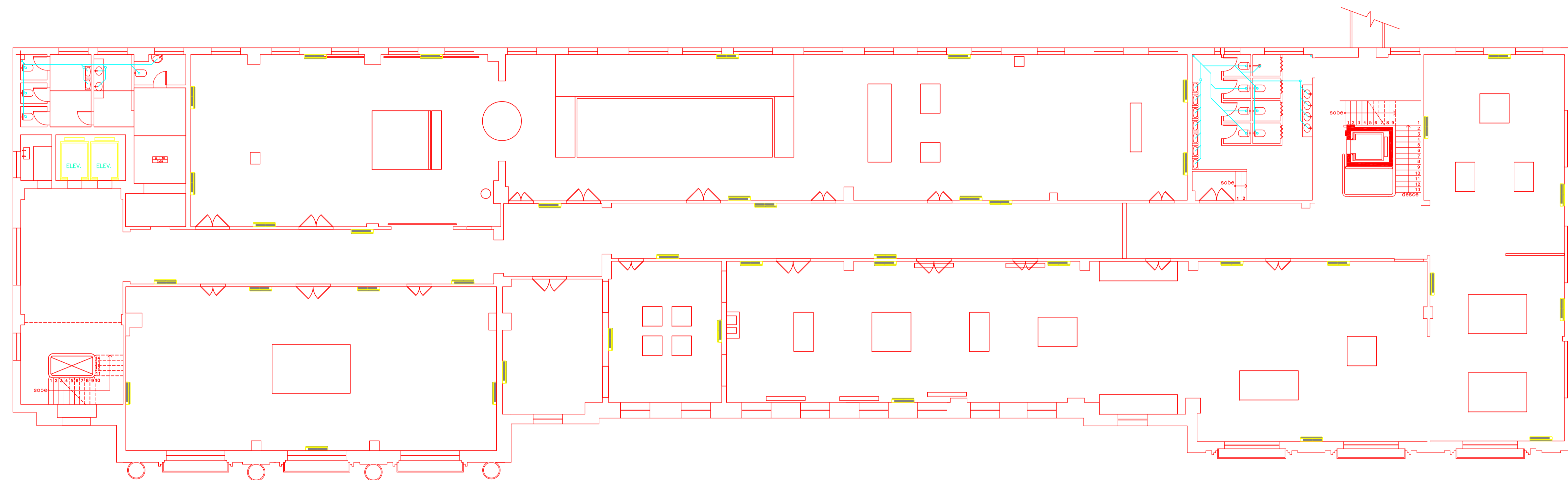
04 PLANTA PAV. SEGUNDO - REDE DE SPRINKLER'S ESC.: 1/125
