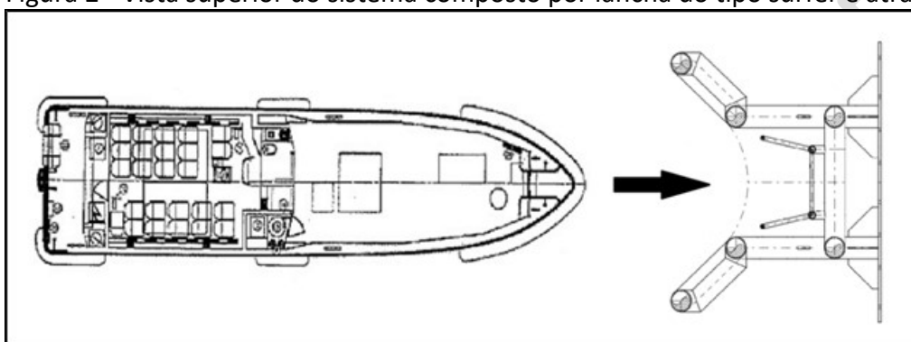
Figura 2 - Vista superior do sistema composto por lança do tipo surfer e atracadouro.
