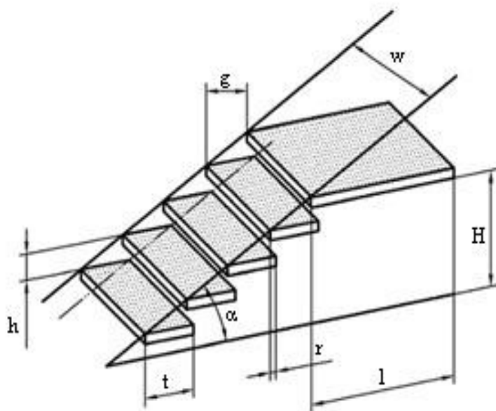
Figura 2: Exemplo de escada sem espelho.
