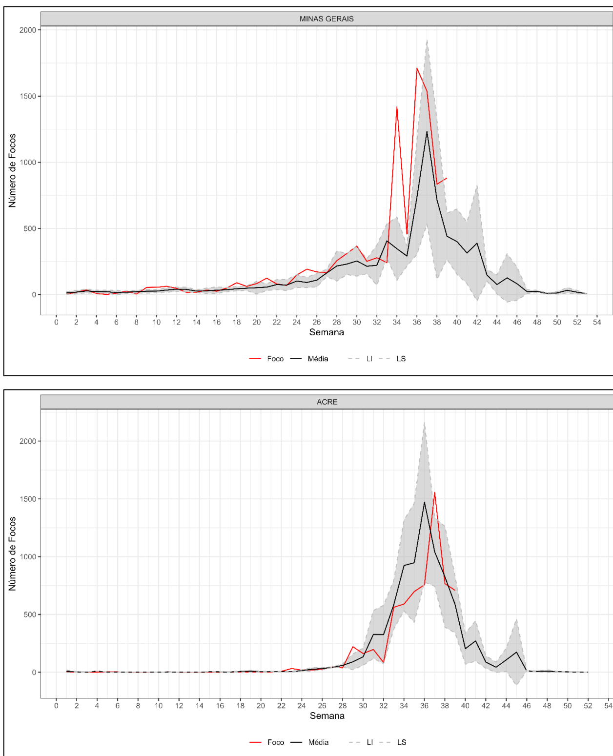
Figura 4. Diagrama de controle dos estados que apresentaram maior número de focos de calor na SE 39.
