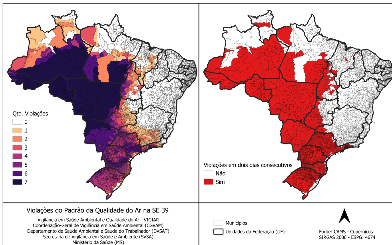
Figura 5. Violações do padrão diário de qualidade do ar nos municípios brasileiros na SE 39 de acordo com as recomendações da OMS ( 15 \mu\text{g}/\text{m}^3 ).
