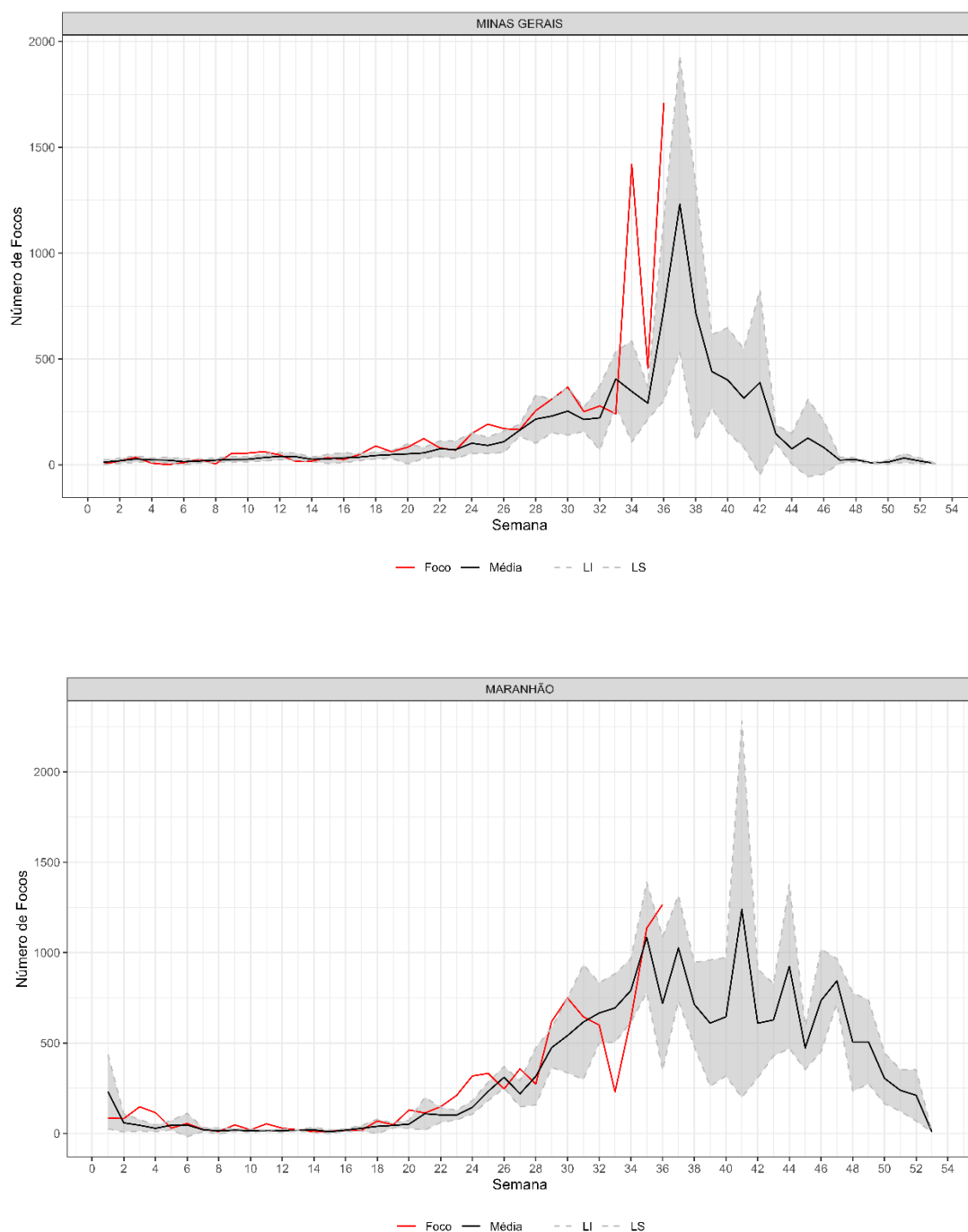
Figura 4. Diagrama de controle dos estados que apresentaram maior número de focos de calor na SE 36.
