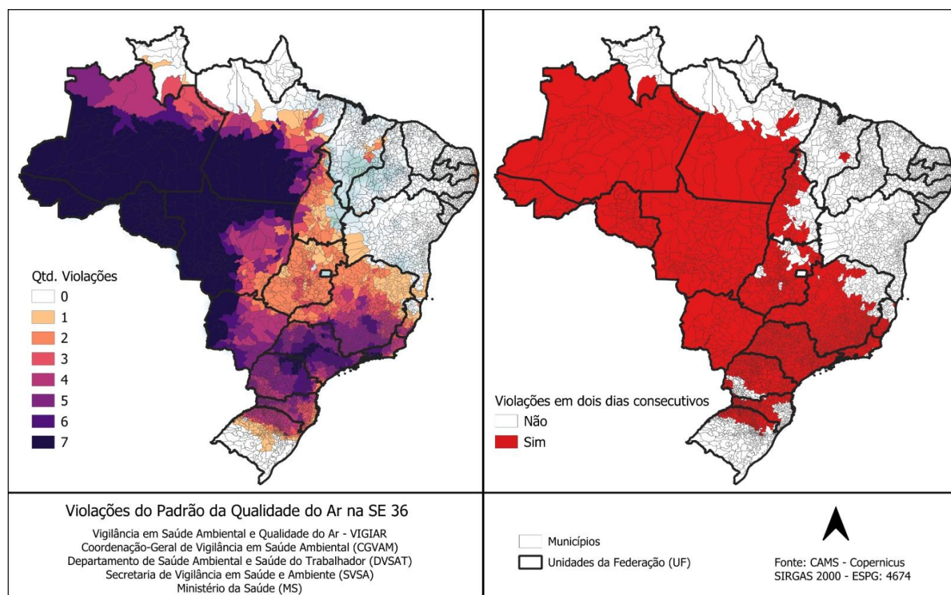
Figura 5. Violações do padrão diário de qualidade do ar nos municípios brasileiros na SE 36 de acordo com as recomendações da OMS ( 15 \mu\text{g}/\text{m}^3 ).
