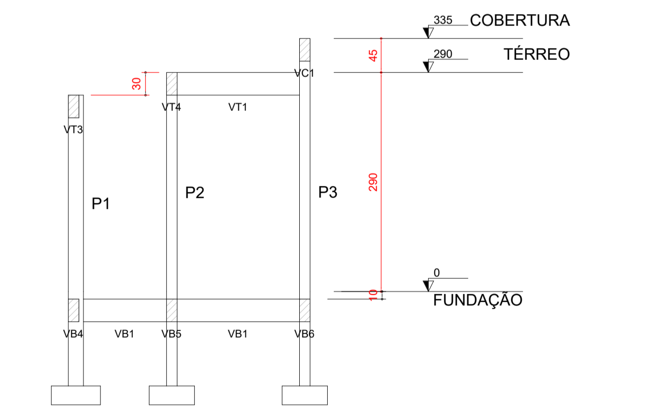
6 CORTE BB ESCALA 1:50
