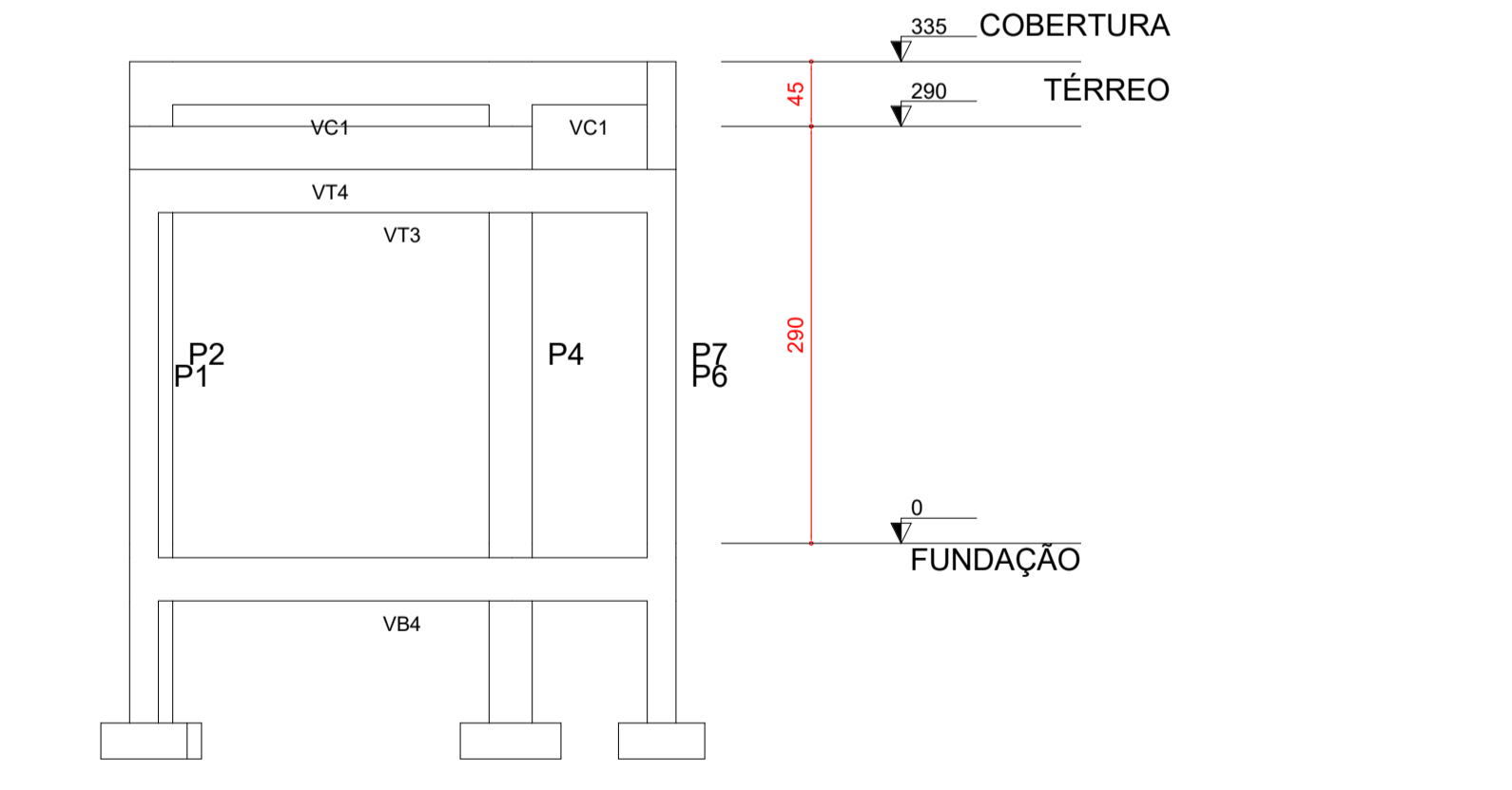
5 CORTE AA ESCALA 1:50
