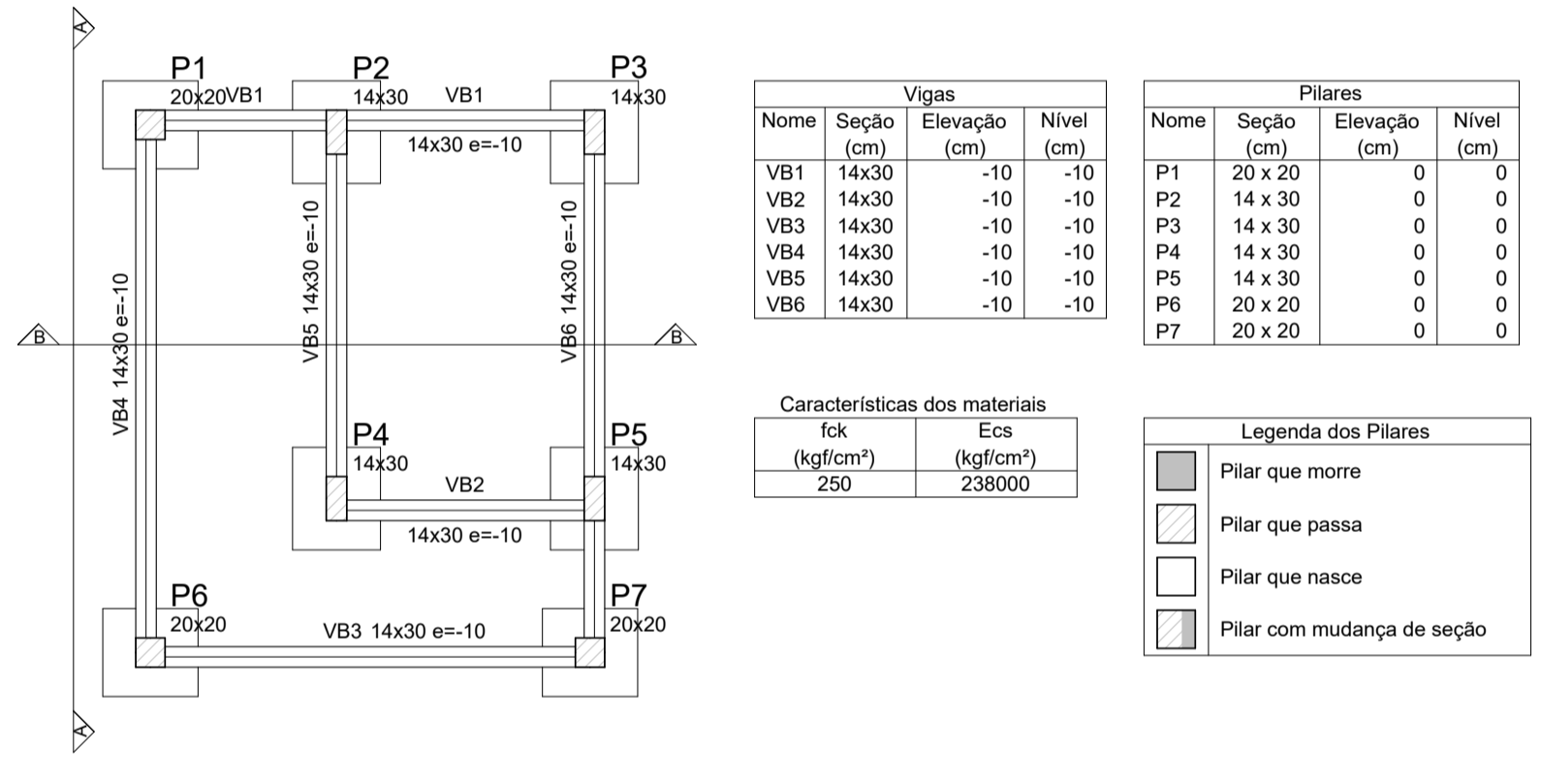
2 PLANTA DE FORMA DA FUNDAÇÃO ESCALA 1:50
