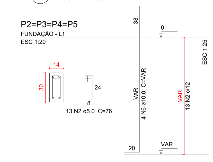
P2=P3=P4=P5 FUNDAÇÃO - L1 ESC 1:20
