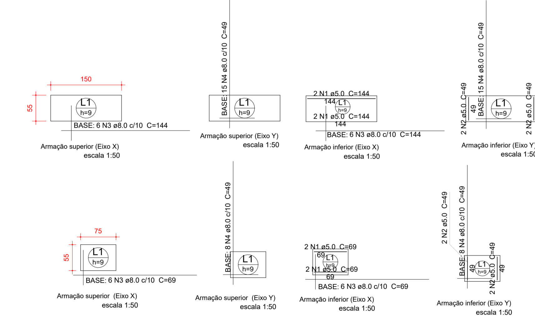
4 ESCOVÓDROMO ESCALA 1:50
