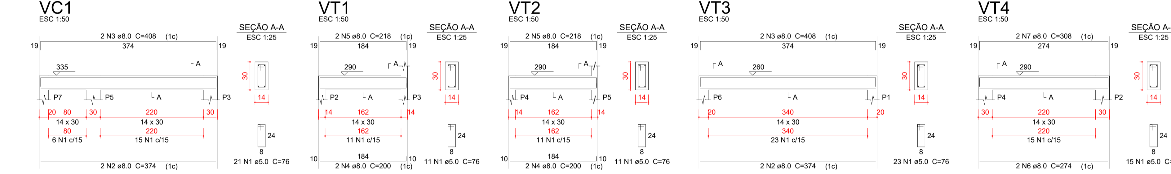
3 DETALHAMENTO VIGAS SUPERIORES ESCALA 1:50
