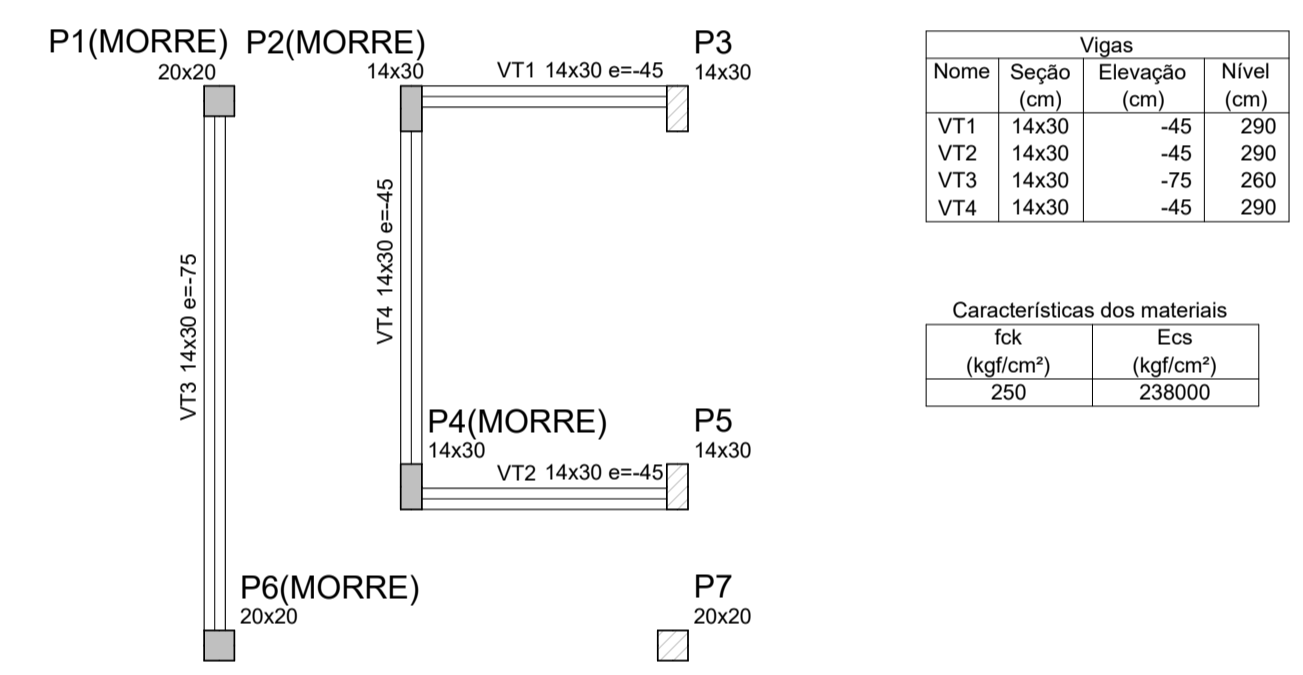
3 PLANTA DE FORMA PAV. TÉRREO ESCALA 1:50
