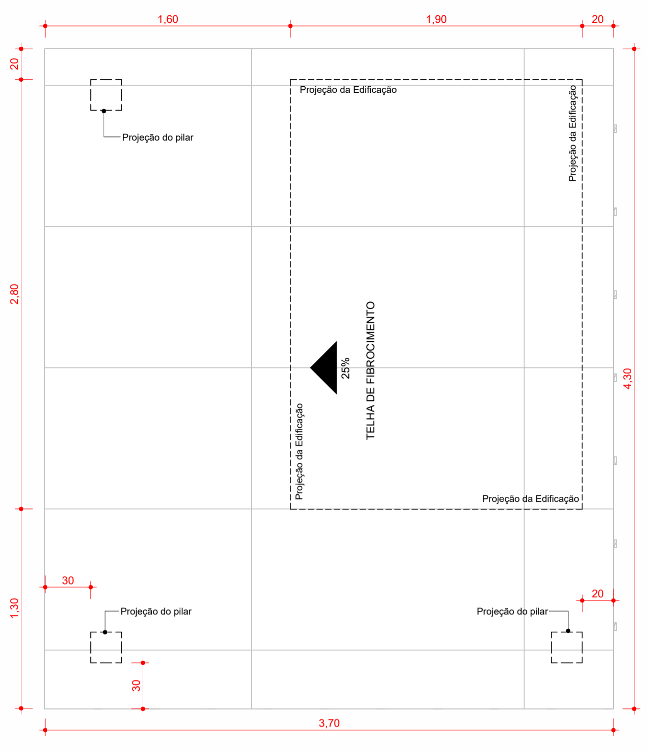
2 COBERTURA ESCALA 1:25
