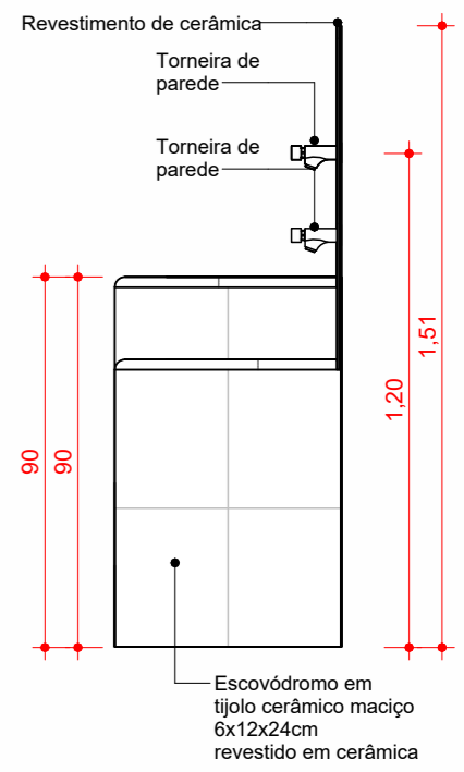
5 Elevação Lateral ESCALA 1 : 20
