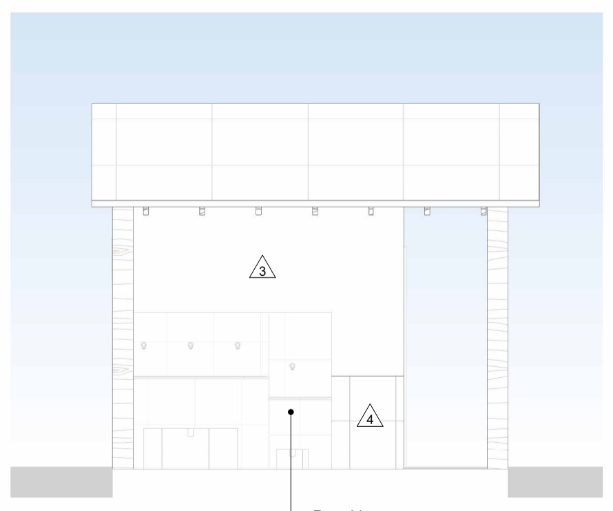
7 FACHADA ESQUERDA ESCALA 1:50
