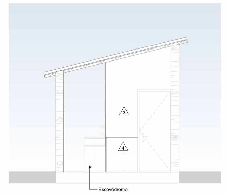
4 FACHADA FRONTAL ESCALA 1:50
