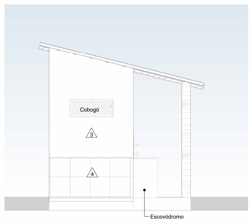
5 FACHADA POSTERIOR ESCALA 1:50
