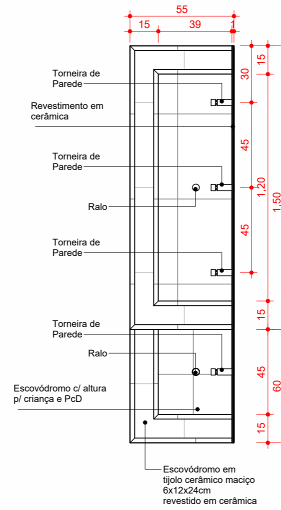
2 Planta de detalhe ESCALA 1 : 20
