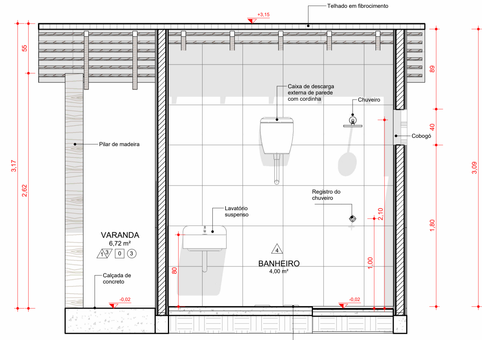
2 CORTE A ESCALA 1:25
