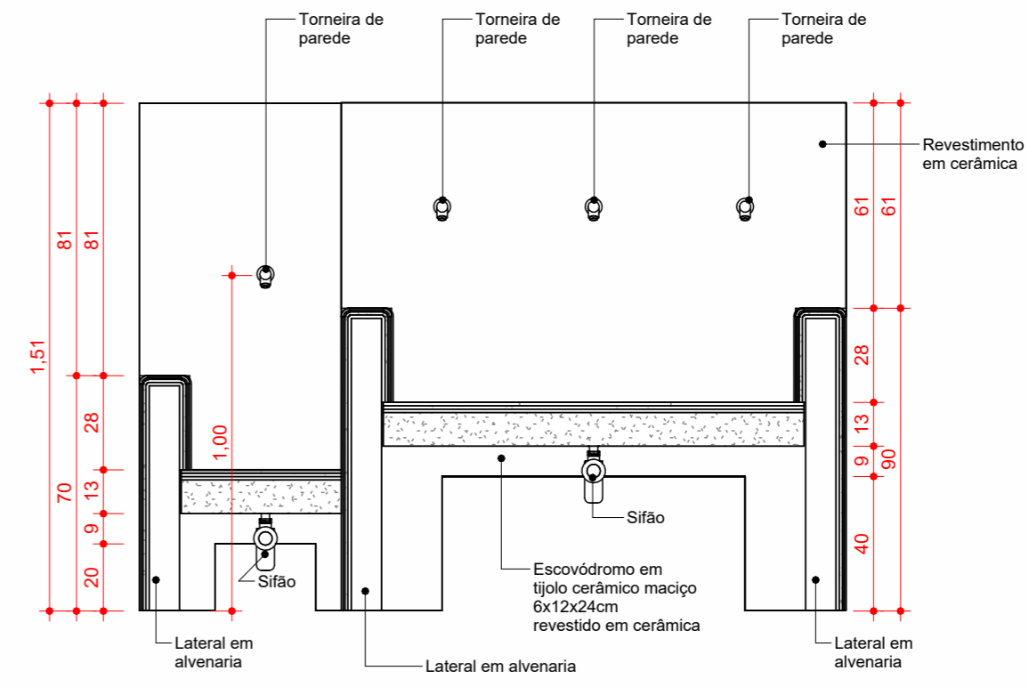
3 Corte ESCALA 1 : 20
