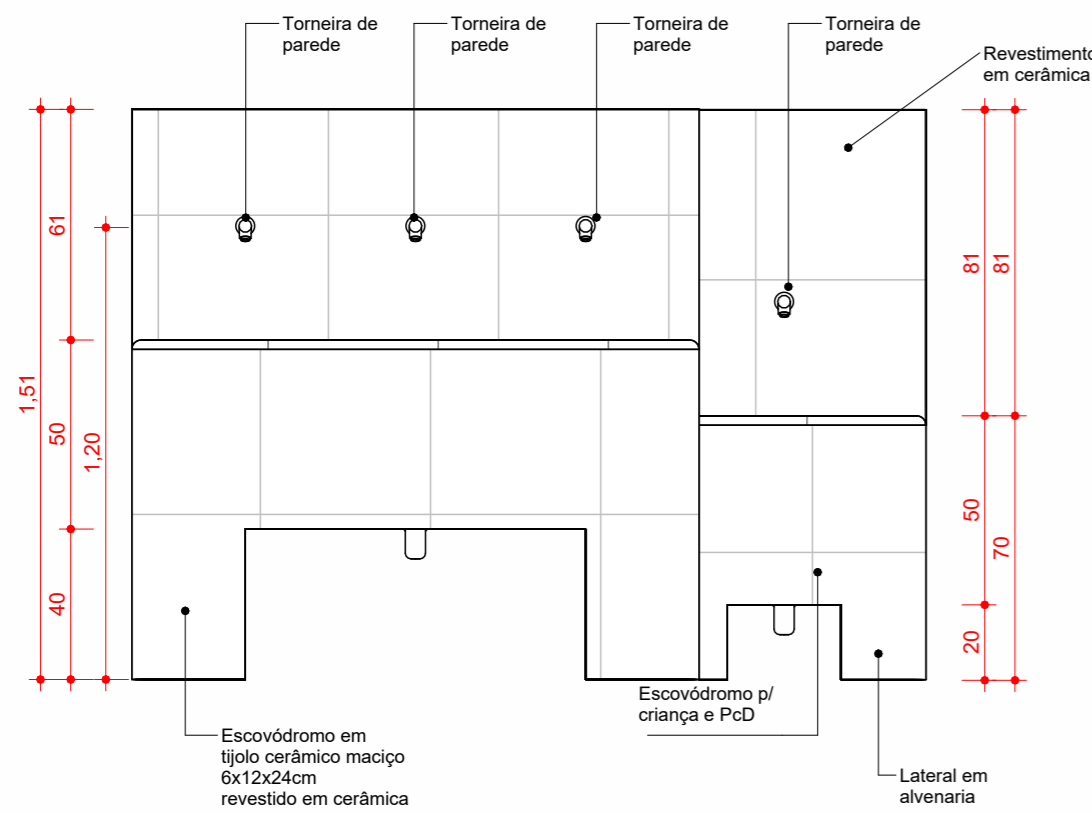
4 Elevação Frontal ESCALA 1 : 20
