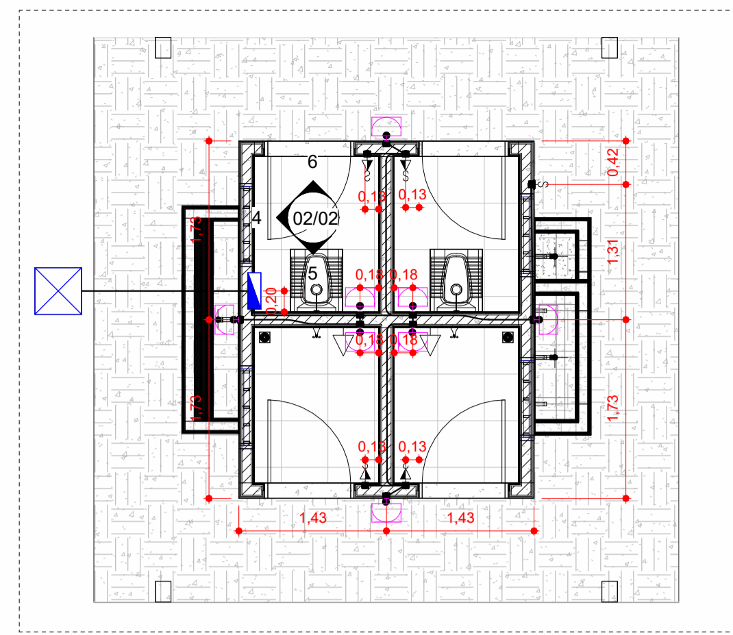
2 PLANTA BAIXA - LOCAÇÃO ESCALA 1:50
