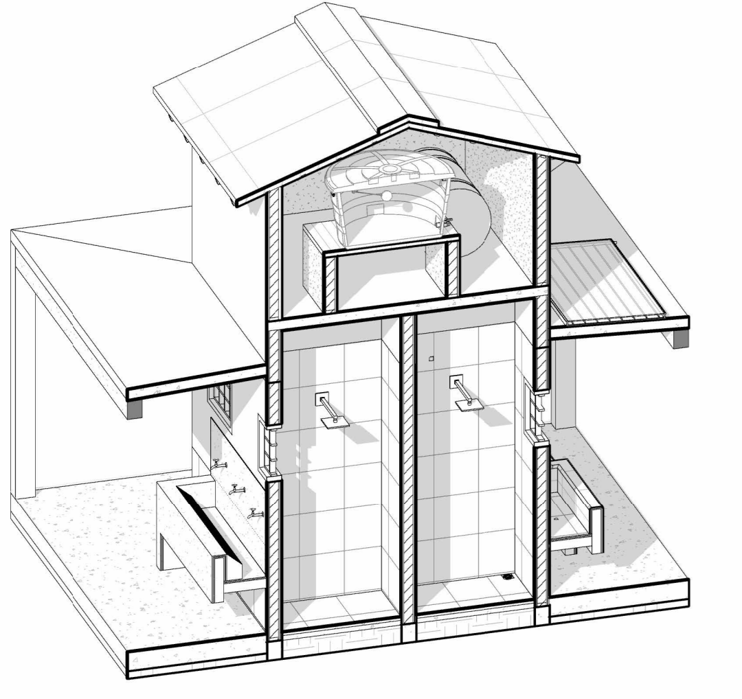
11 CORTE PERSPECTIVA - 03 ESCALA
