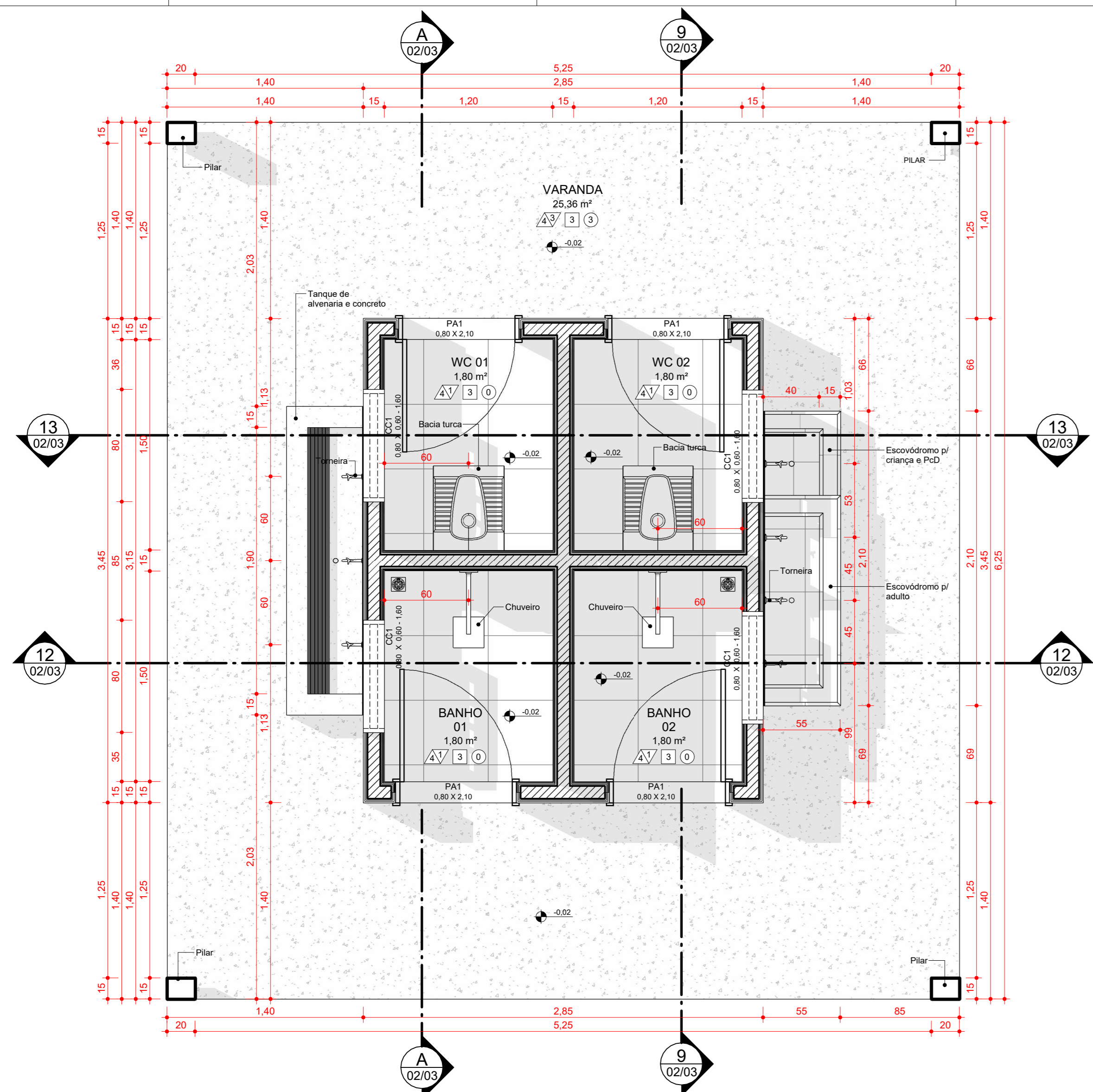
01 TERREO - CONSTRUÇÃO NOVA ESCALA 1:25
