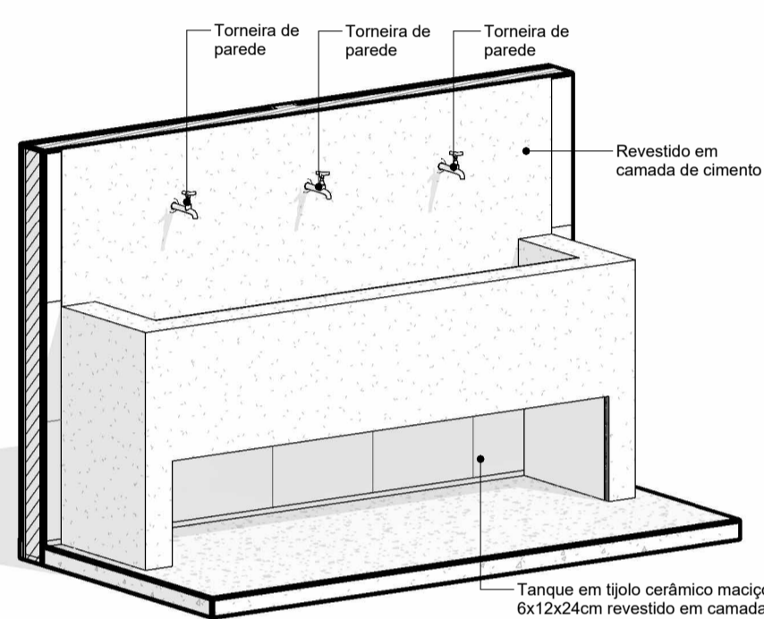
8 PERSPECTIVA TANQUE ESCALA
