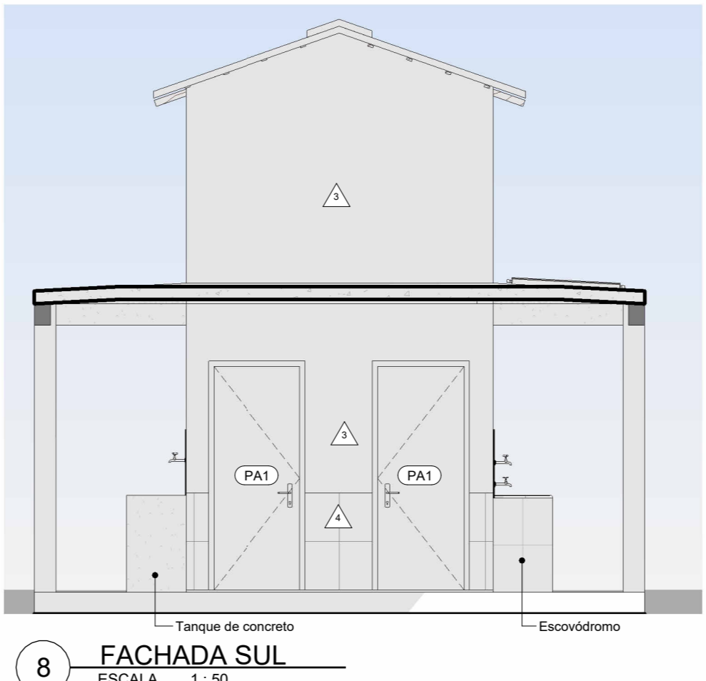
8 FACHADA SUL ESCALA 1:50
