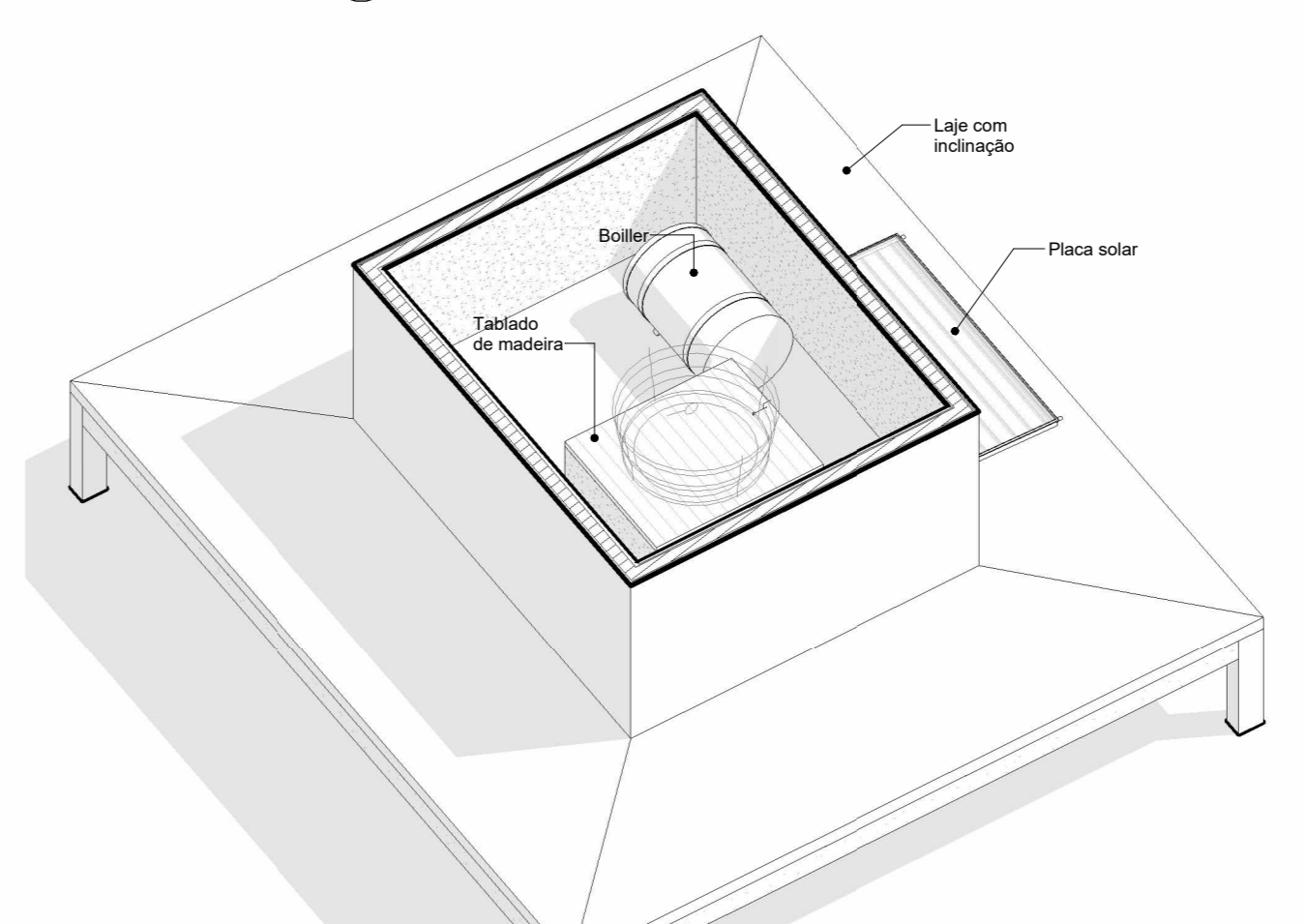
14 PERSPECTIVA COBERTURA ESCALA
