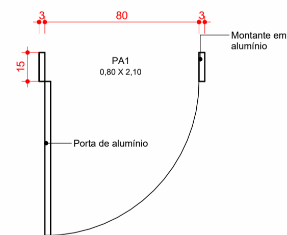
14 Planta de detalhe ESCALA 1:20
