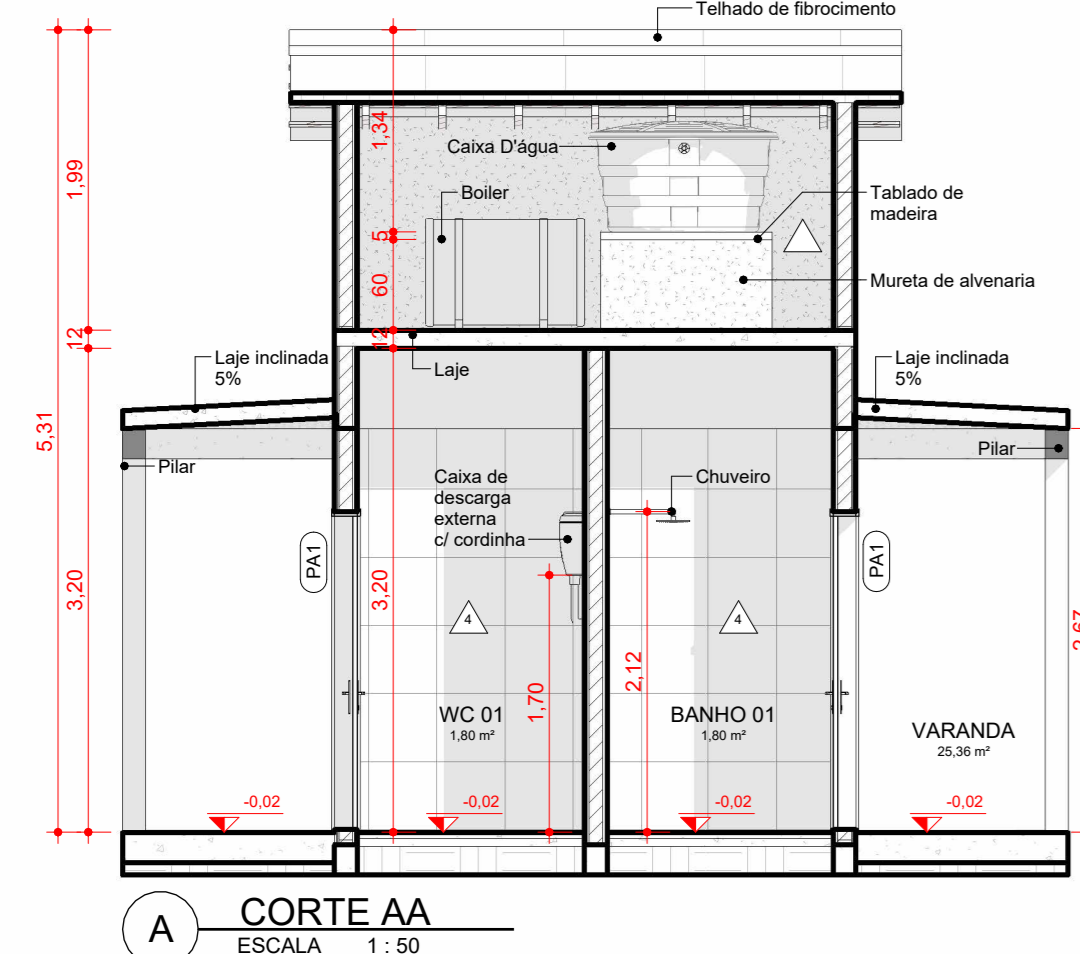
A CORTE AA ESCALA 1:50
