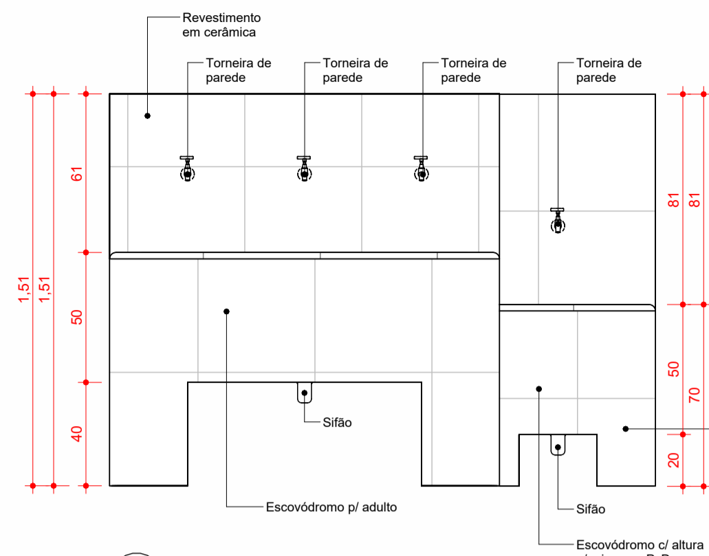
4 Elevação Frontal ESCALA 1:20
