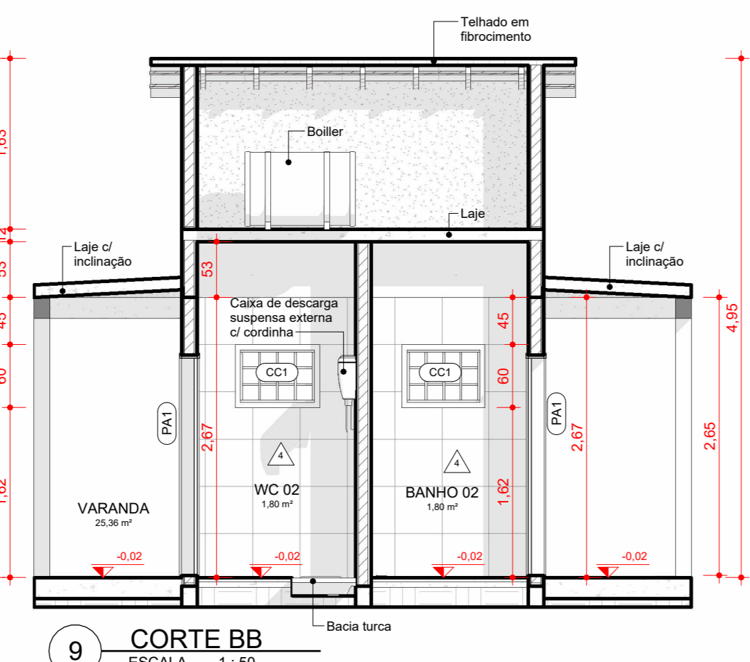
9 CORTE BB ESCALA 1:50
