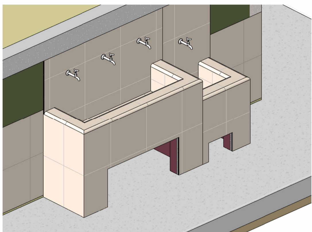
6 VISTA 3D 1 PIAS EXTERNAS ESCALA
