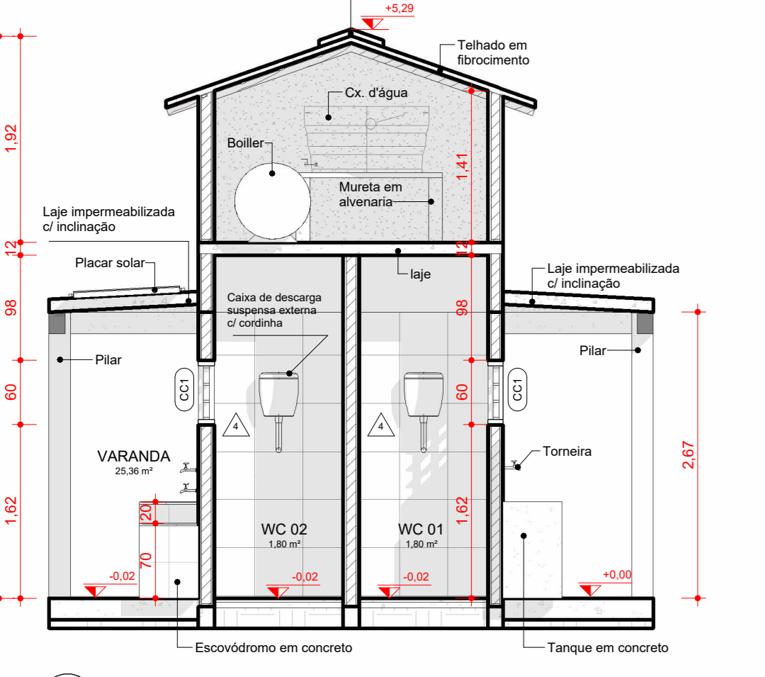
13 CORTE DD ESCALA 1:50
