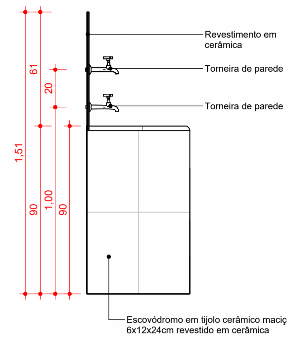
5 Vista lateral ESCALA 1:20
