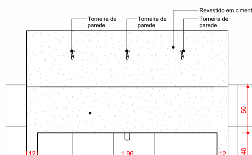
9 01. TÉRREO - DET. TANQUE ESCALA 1:25
