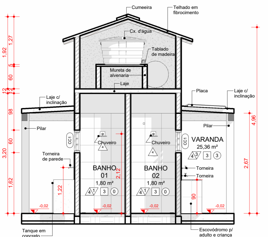
12 CORTE CC ESCALA 1:50
