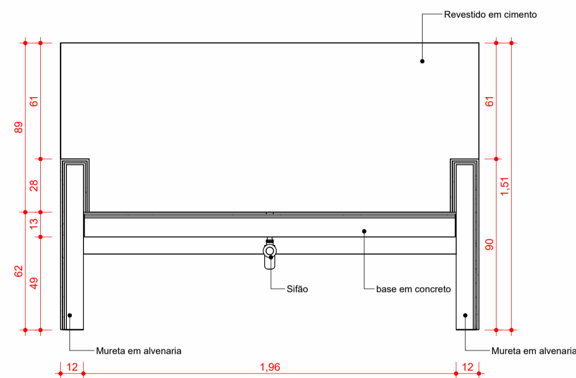
21 CORTE ESCALA 1:20
