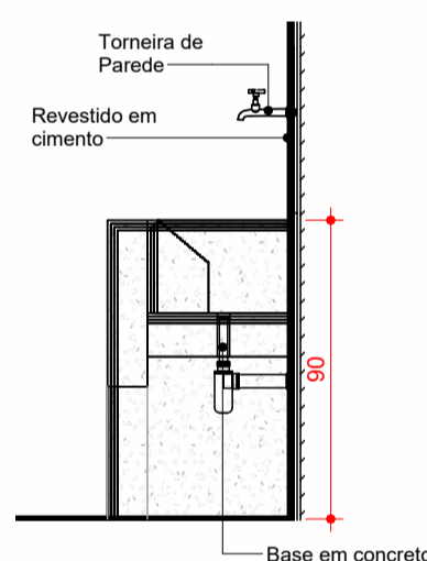
10 VISTA LATERAL TANQUE ESCALA 1:25
