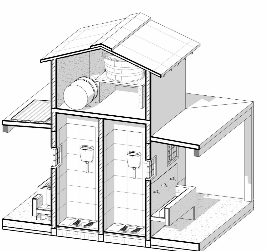
10 CORTE PERSPECTIVA - 02 ESCALA
