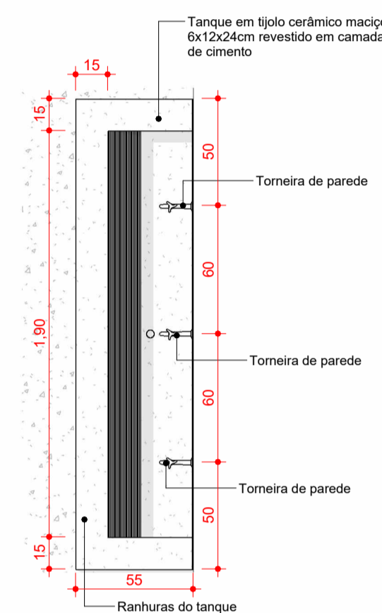
9 01. TÉRREO - DET. TANQUE ESCALA 1:25
