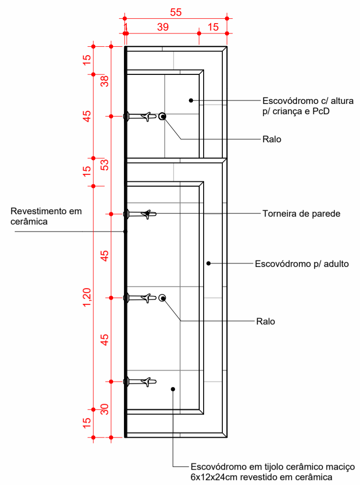
2 Planta de detalhe ESCALA 1:20
