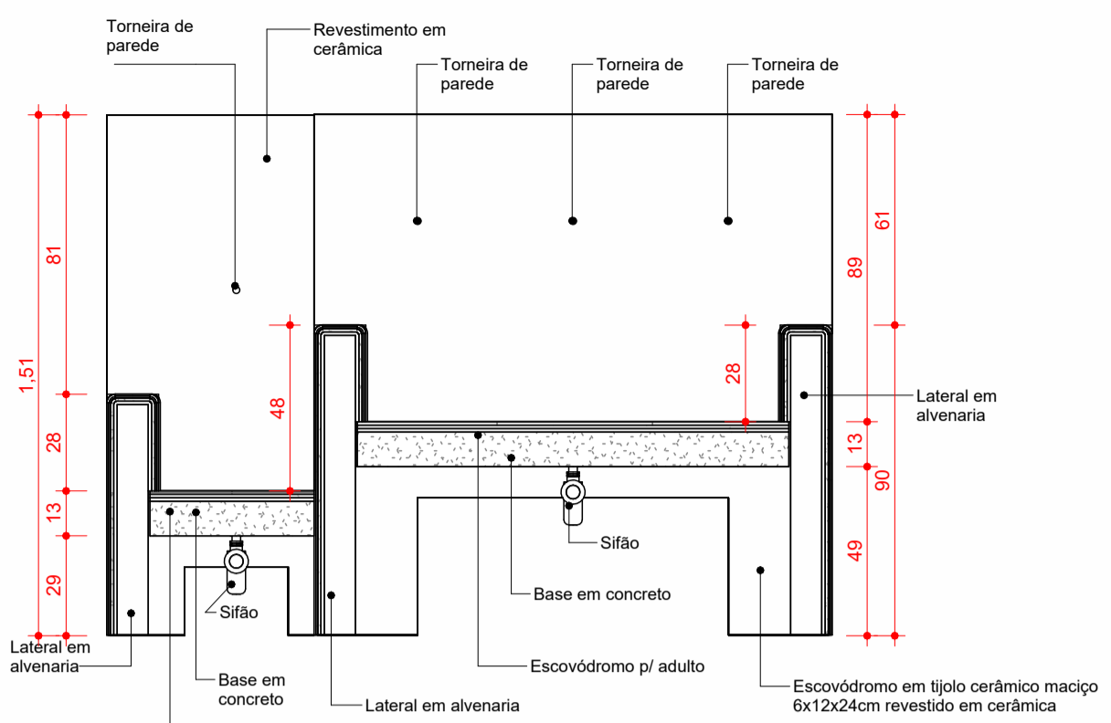
3 Corte ESCALA 1:20
