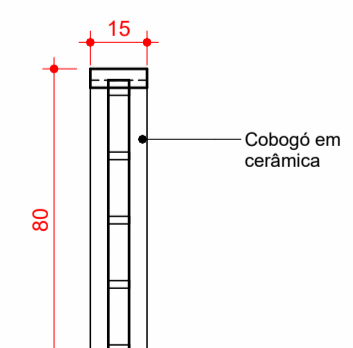
18 Planta de detalhe ESCALA 1:20
