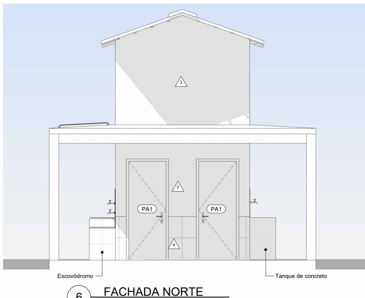
6 FACHADA NORTE ESCALA 1:50
