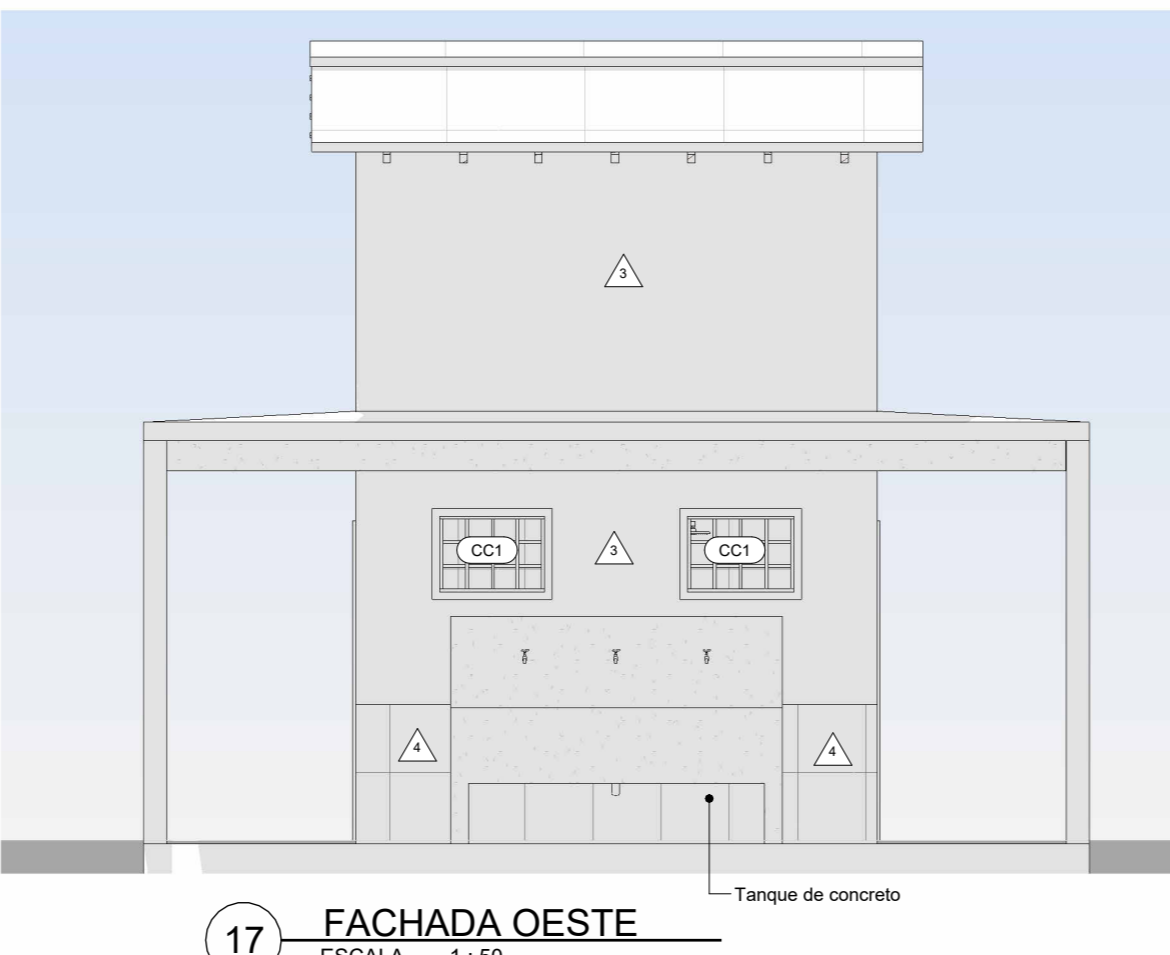
17 FACHADA OESTE ESCALA 1:50
