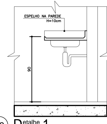
09 Detalhe 1 Esc.: 1:25
