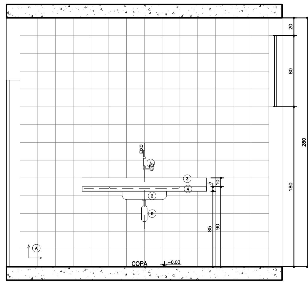
08 Seção AA' Amb. 04 - Copa Esc.: 1:25
