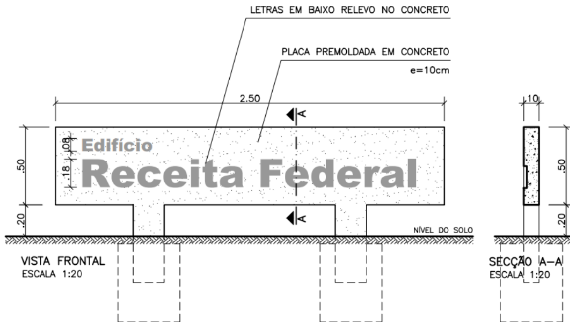
Projeto – Placa de Identificação Edifício-Sede
