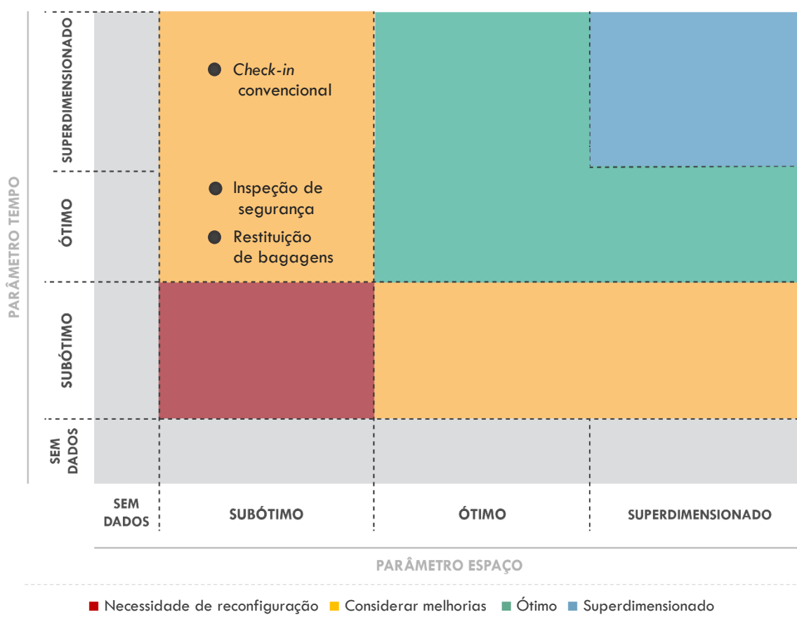
Figura 9 – Diagrama de espaço-tempo para o nível de serviço oferecido no Aeroporto de Governador Valadares Fonte: IATA (2014) e dados obtidos do questionário aplicado ao operador aeroportuário. Elaboração: LabTrans/UFSC (2016)
