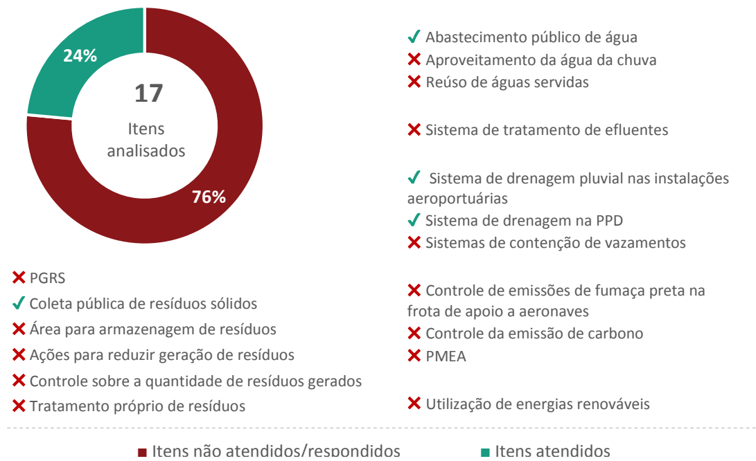
Gráfico 26 – Aspectos ambientais: Aeroporto de Governador Valadares Fonte: Dados obtidos do questionário aplicado ao operador aeroportuário. Elaboração: LabTrans/UFSC (2016)
