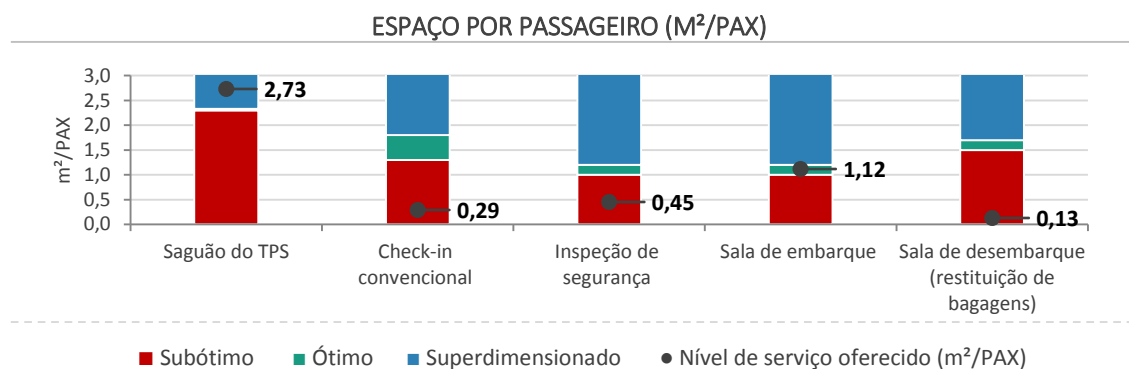
Gráfico 13 – Nível de serviço oferecido pelos componentes em relação ao parâmetro “espaço por passageiro” Fonte: Dados obtidos do questionário aplicado ao operador aeroportuário. Elaboração: LabTrans/UFSC (2016)
