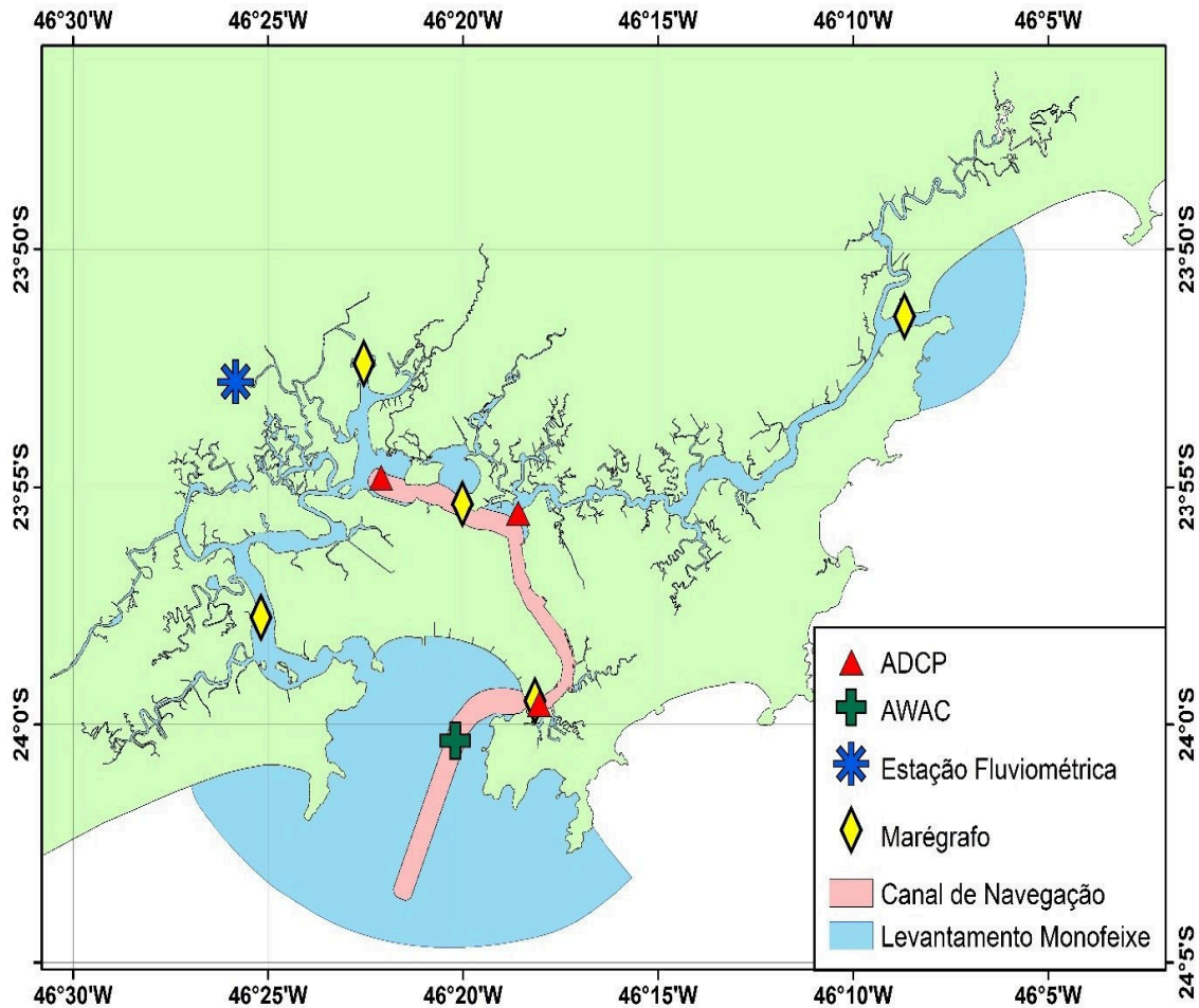
Figura 02. Localização das estações maregráficas e fluviométrica, ADCP e AWAC.
