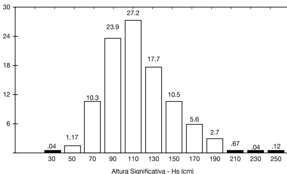
Figura 20 - Histograma da altura significativa
