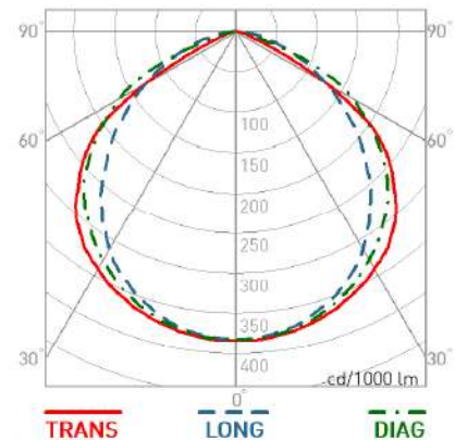
Curva de distribuição Fotométrica Ilustrativa - Ref. modelo Itaim Arcos.
