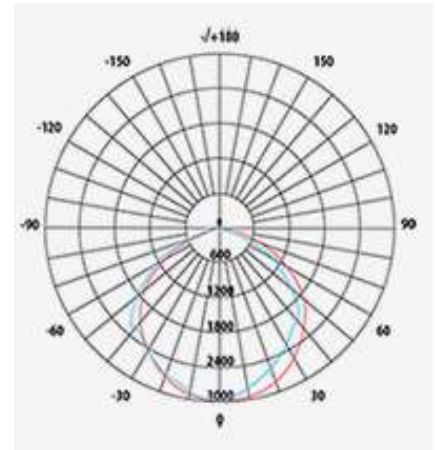
Curva de distribuição Fotométrica Ilustrativa - Ref. modelo Brilia smart projetor.
