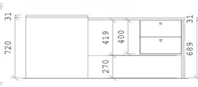
06-Corte Lateral Direito
