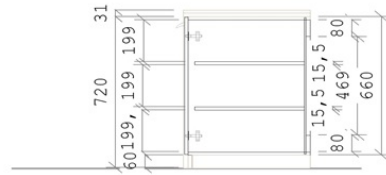
06-Corte Lateral Direito
