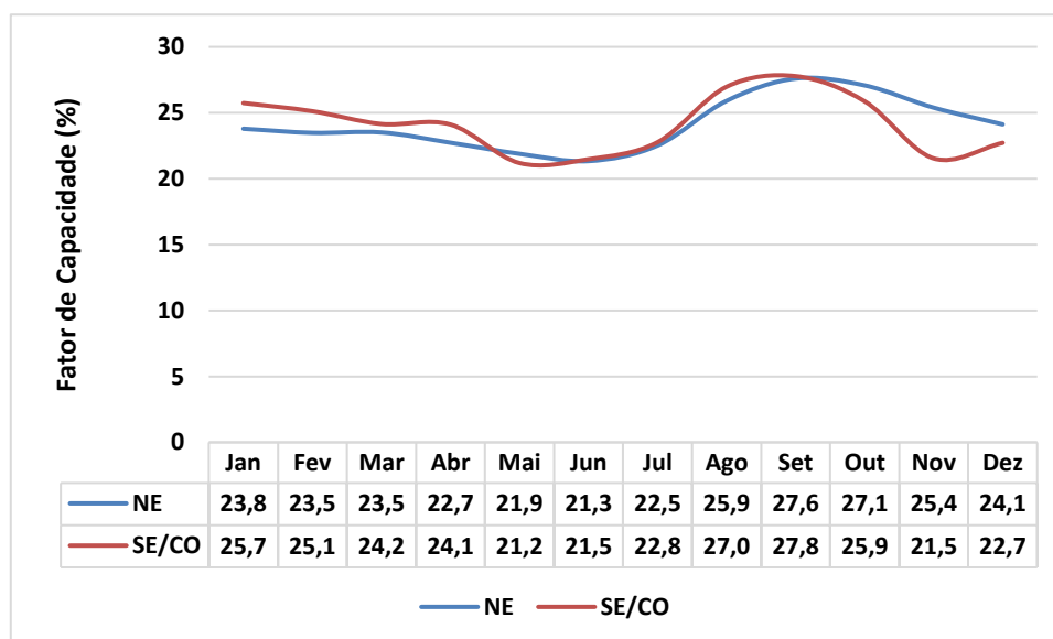
Figura 19 – Fotovoltaica Flutuante: Fator de capacidade mensal por subsistema
