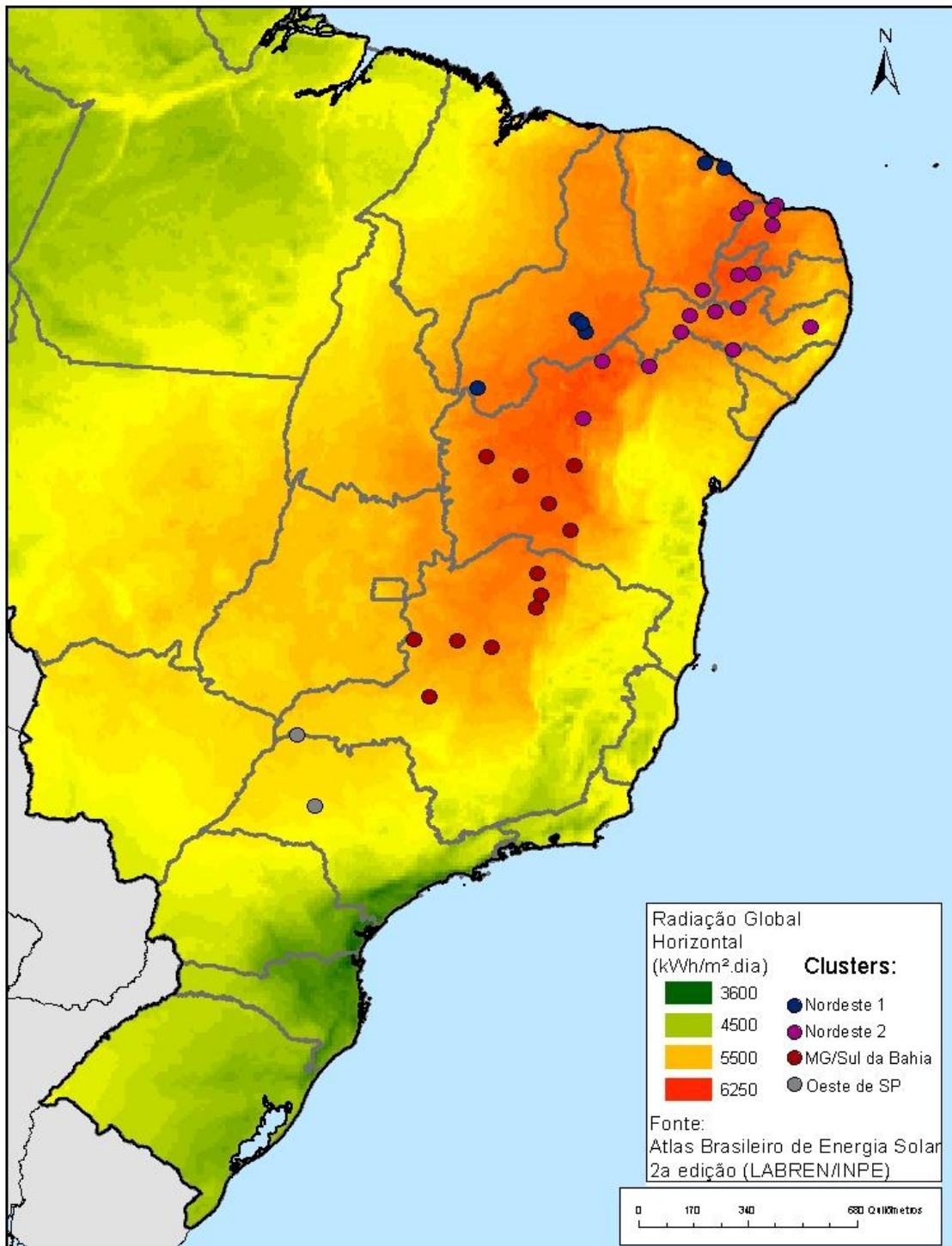
Figura 8 – Divisão por clusters dos pontos simulados para solar fotovoltaica
