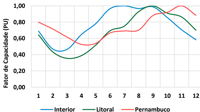
Figura 11 – Regiões do Nordeste: Comportamento Mensal
