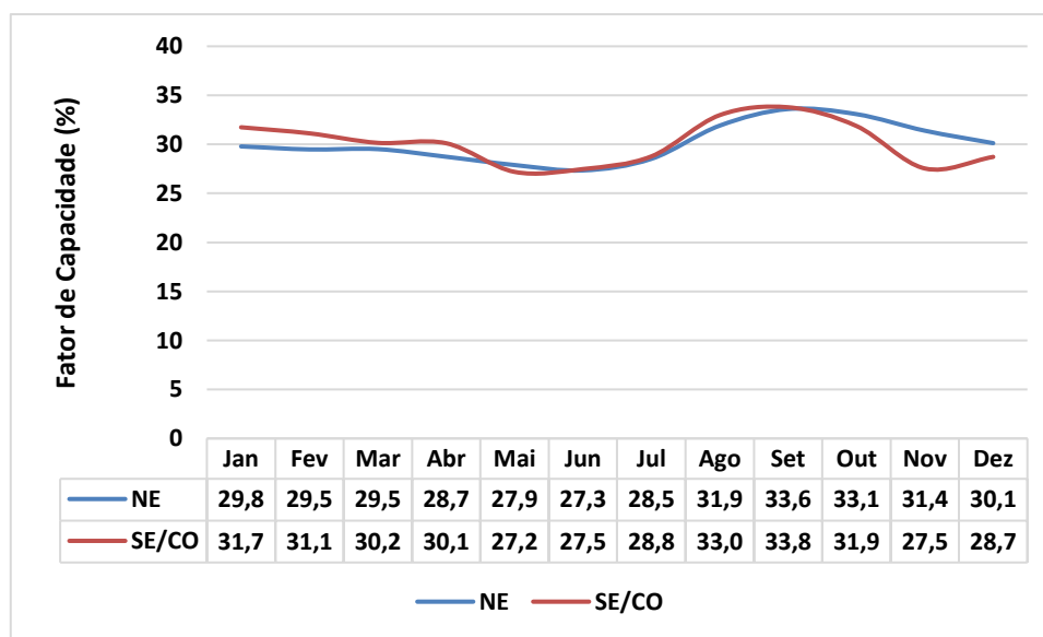
Figura 18 – Fotovoltaica: Fator de capacidade mensal por subsistema
