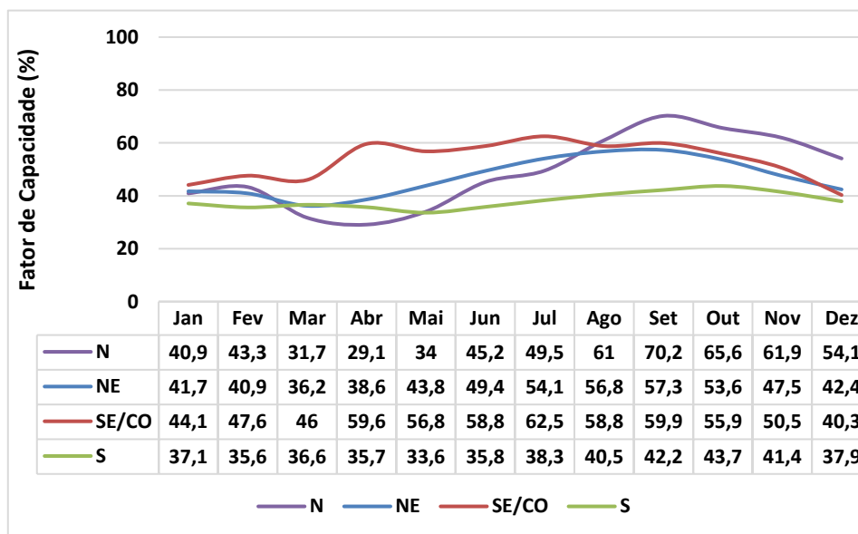
Figura 20 – Eólica onshore : Fator de capacidade mensal por subsistema
