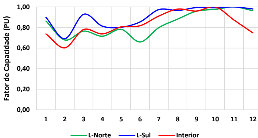
Figura 16 – Regiões do Sul: Comportamento Mensal
