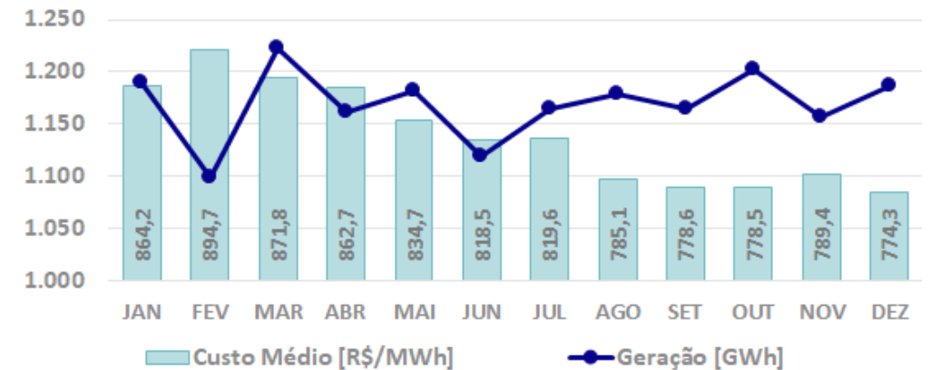
Custo Médio [R$/MWh] x Geração [MWh]
