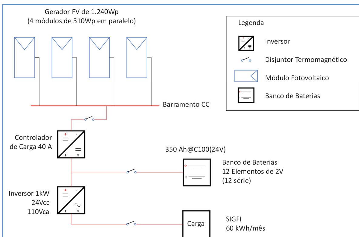
Figura 3 – Exemplo de diagrama unifilar
