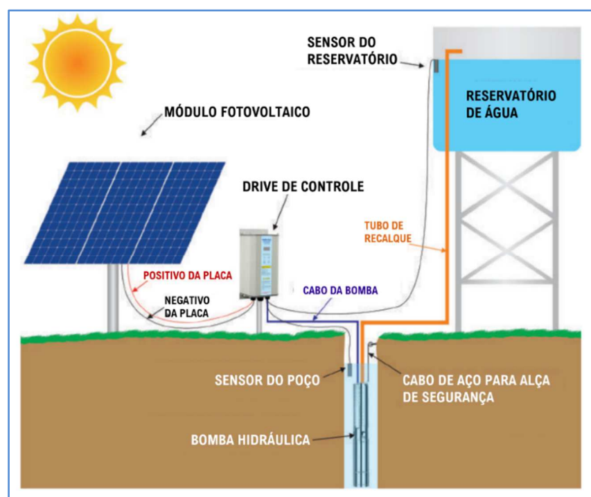
Figura 7 – Diagrama esquemático de um SBFV (Fonte: Página da Internet 1 )
