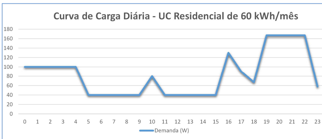
Figura 2 – Exemplo de Curva de Carga Residencial
