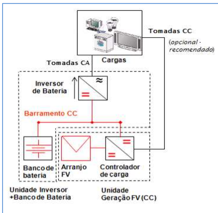
Figura 2 - Configuração SIGFI
