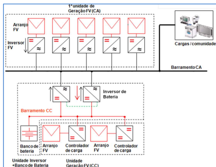
Figura 6 – Configuração MIGDI CA/CC
