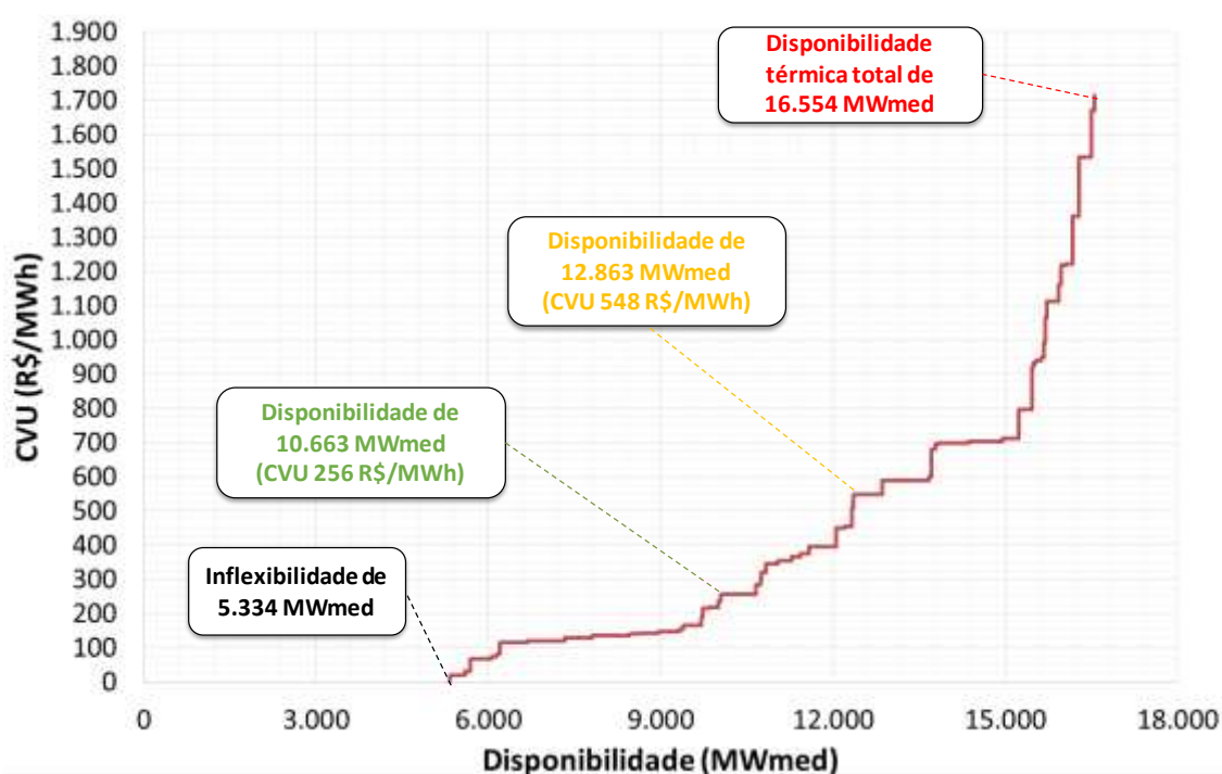
Figura 233 - Custo Variável Unitário (CVU) das Usinas Térmicas
