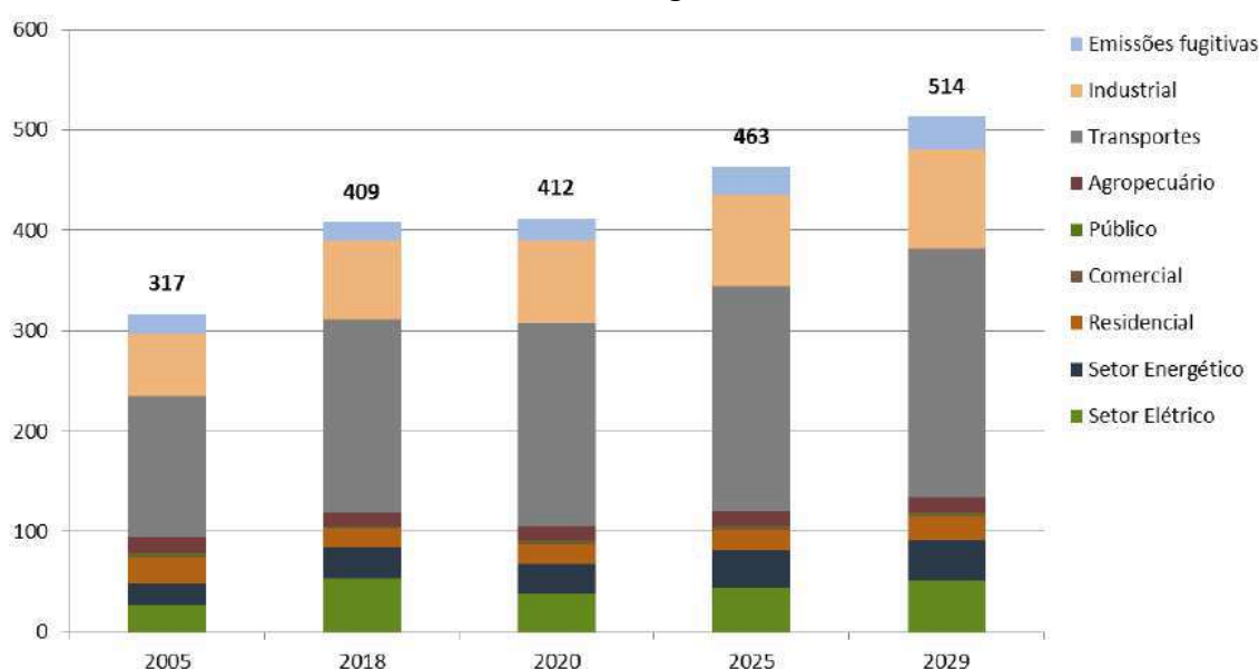
Figura 7 - Evolução da participação setorial nas emissões de GEE pela produção e uso de energia
