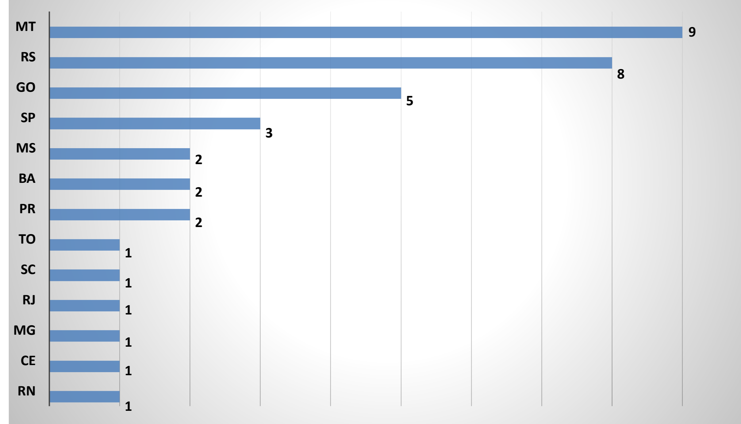
Número de Usinas Produtoras de Biodiesel com Selo Combustível Social por UF - Última atualização em 12/01/2017
