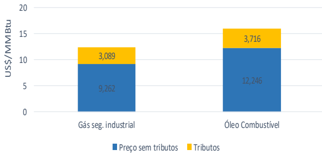
Comparativo de preços entre gás natural para segmento industrial (20.000 m³/d) e óleo combustível em São Paulo - janeiro/2019
