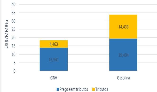
Comparativo de preços entre GNV e gasolina em São Paulo - agosto/2017
