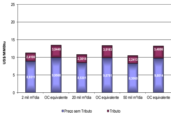
Comparativo de Preços entre Gás Natural Industrial e OCA1 na Bahia - agosto/2016
