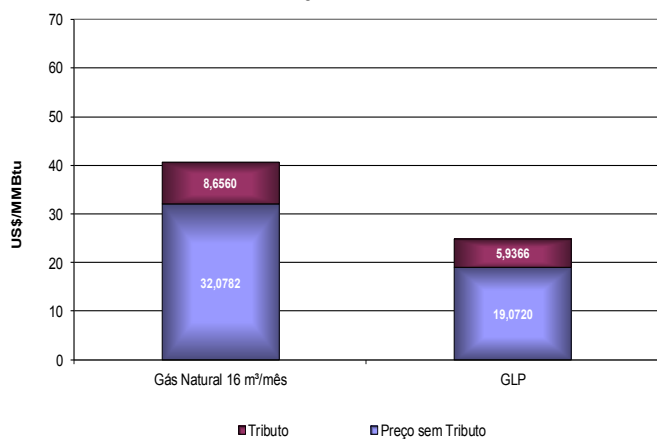
Comparativo de Preços entre Gás Natural Residencial e GLP no Rio de Janeiro - agosto/2016
