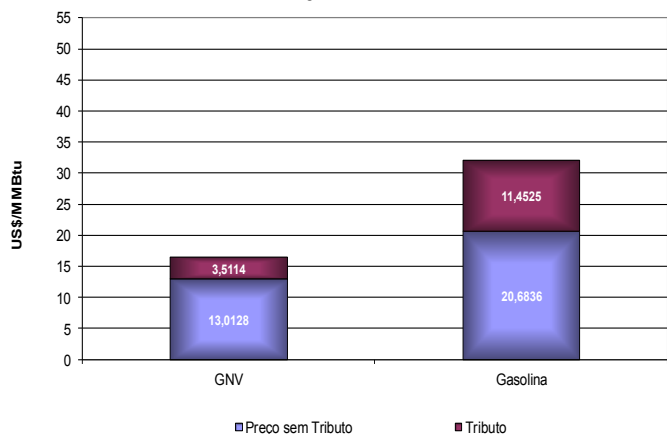
Comparativo de Preços entre Gás Natural Veicular e Gasolina em São Paulo - agosto/2016
