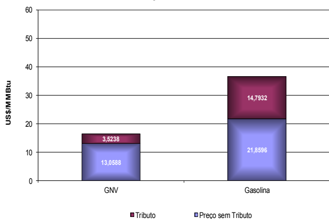
Comparativo de Preços entre Gás Natural Veicular e Gasolina no Rio de Janeiro - agosto/2016
