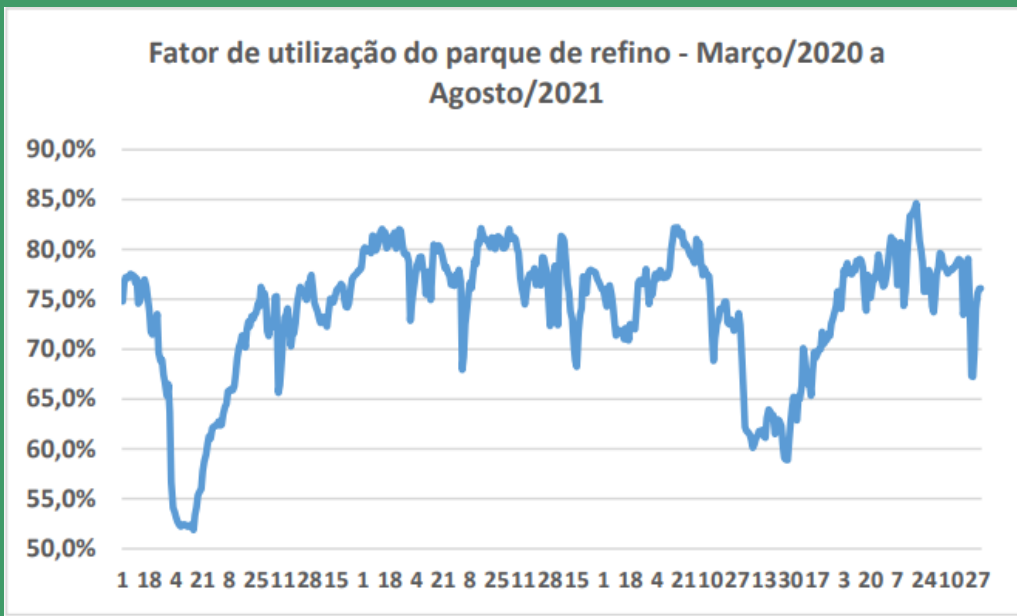
Fator de utilização global das refinarias do sistema Petrobras.
