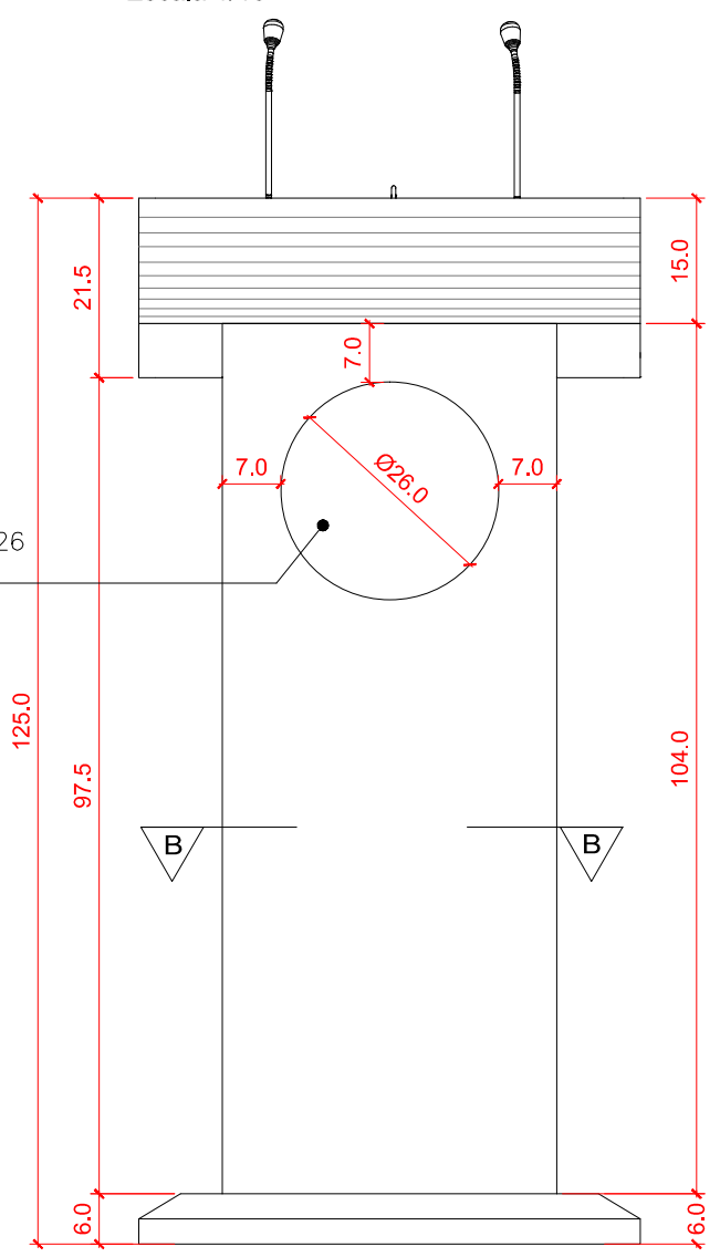
VISTA FRONTAL Escala 1/10
