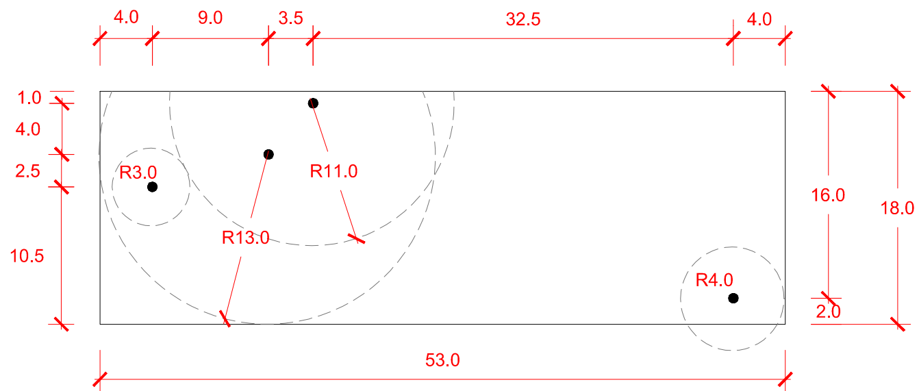
MARCAÇÃO CURVATURAS 01 Escala 1/5
