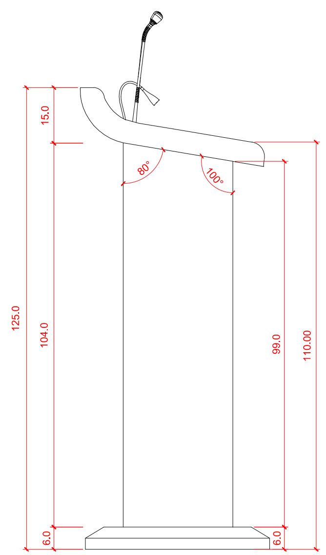
VISTA LATERAL Escala 1/10
