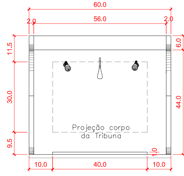
VISTA SUPERIOR Escala 1/10
