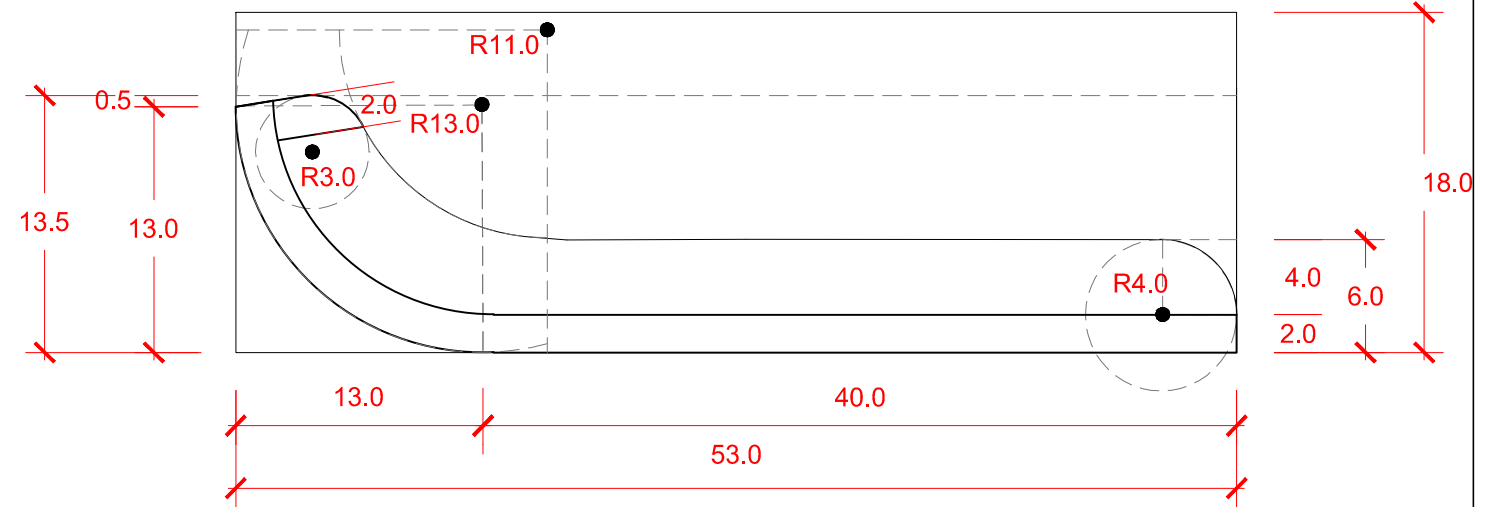
MARCAÇÃO CURVATURAS 02 Escala 1/5
