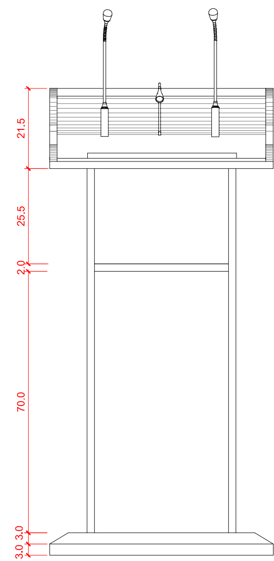
VISTA POSTERIOR Escala 1/10
