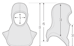
Figura 7 - medidas do capuz tipo balaclava
