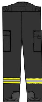
Fig.4 - vista traseira da calça de proteção
