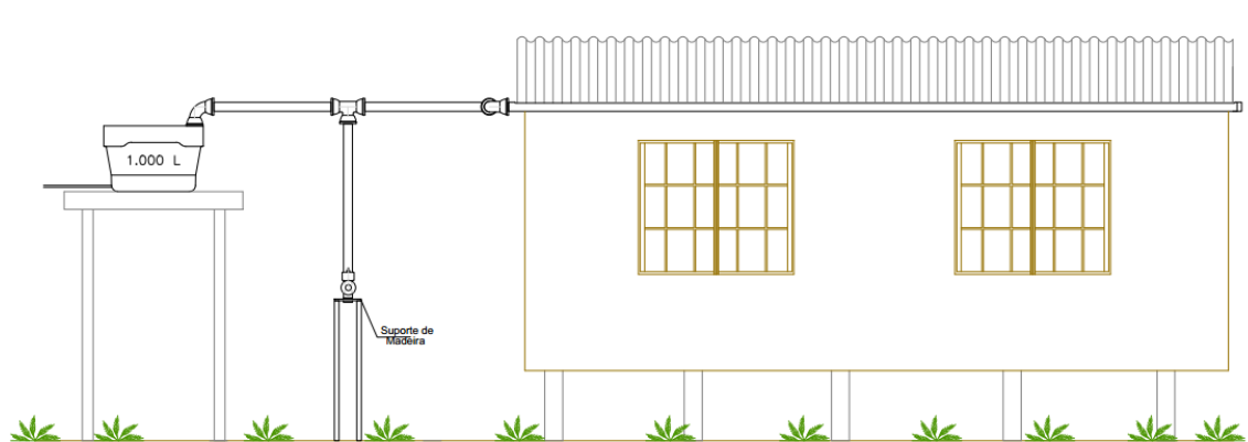
Figura 1: Desenho com os itens que compõem o componente de captação da água de chuva.
