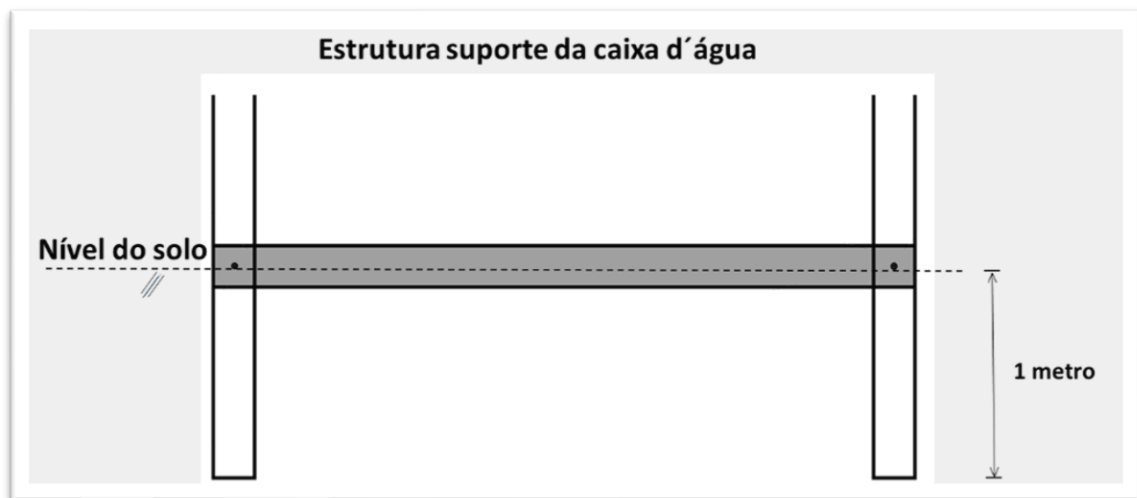
Figura 5: Esquema da locação em relação ao solo da estrutura de amarração construída na base da estrutura que dá suporte a caixa de 5.000 litros.
