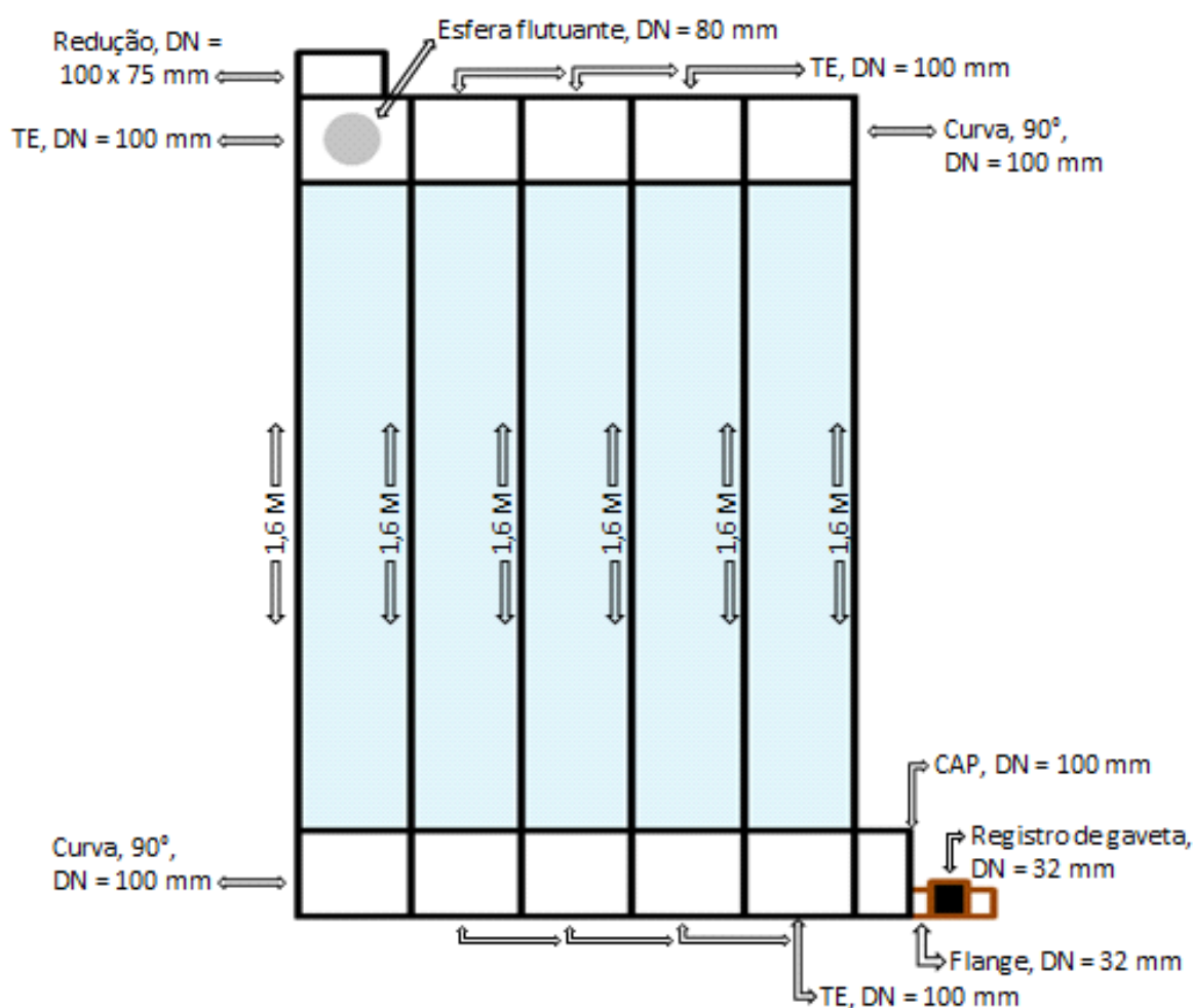
Figura 13: Modelo do dispositivo DesvUFPE para proteção da qualidade da água
