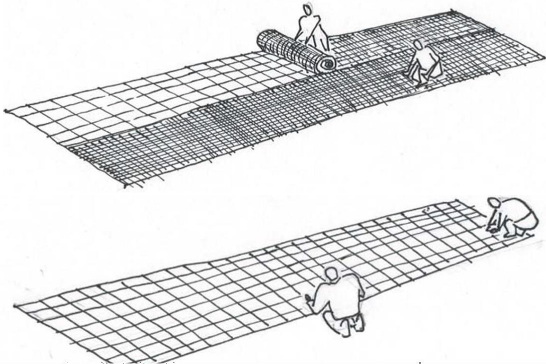
Figura 4: Ilustração do processo de confecção da armadura da parede da cisterna
