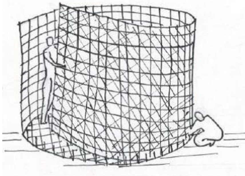
Figura 5: Ilustração do processo de confecção da armadura da parede da cisterna
