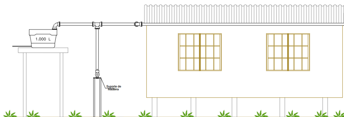
Figura 2: Desenho com os itens que compõem o componente de captação da água de chuva.
