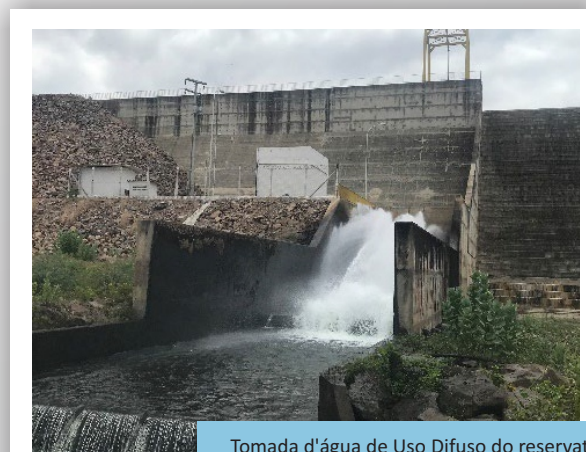
Tomada d'água de Uso Difuso do reservatório Porcos, WBS 1113, Trecho II, Eixo Norte do PISF.
