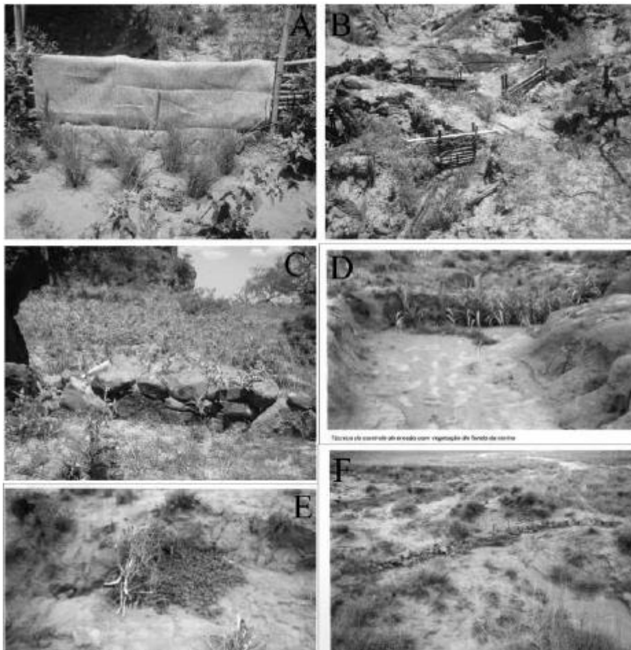
Técnicas de controle de erosão hídrica em áreas degradadas. (A/ B) Paliçadas de Bambu, (C) Barreira de rochas, (D) Barreira vegetal (E) Barreira física com galhos e (F) Barreira de rochas. Fonte: Verdum, Vieira e Caneppele (2016).
