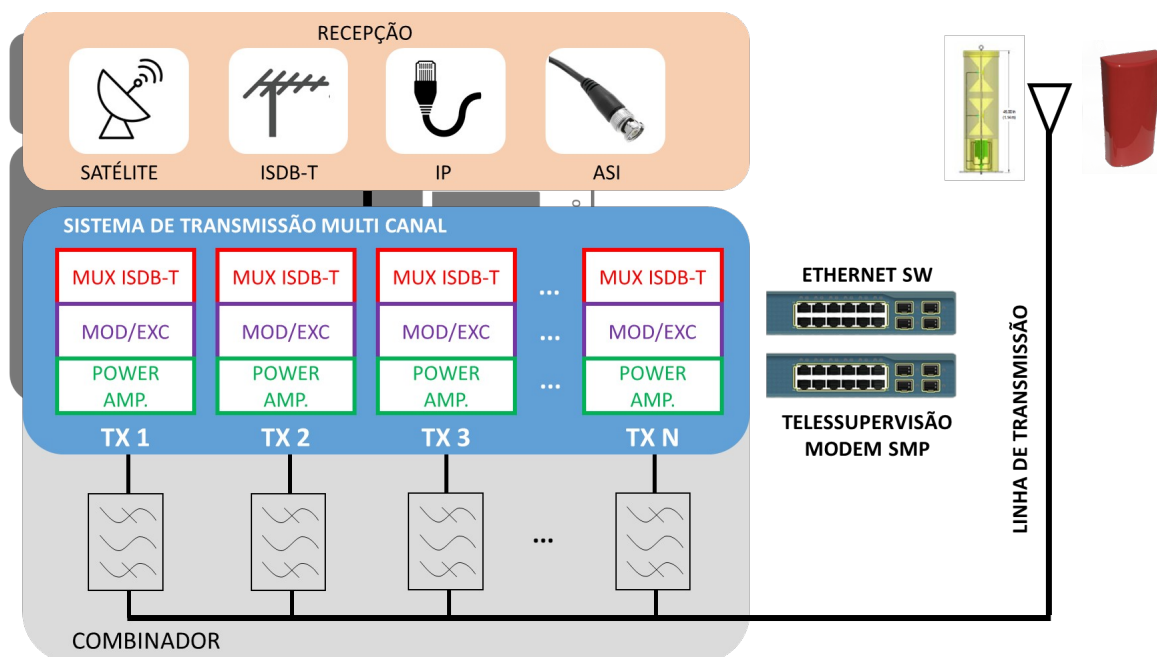
Figura 1: Sistema de Transmissão Multicanal (STM)
