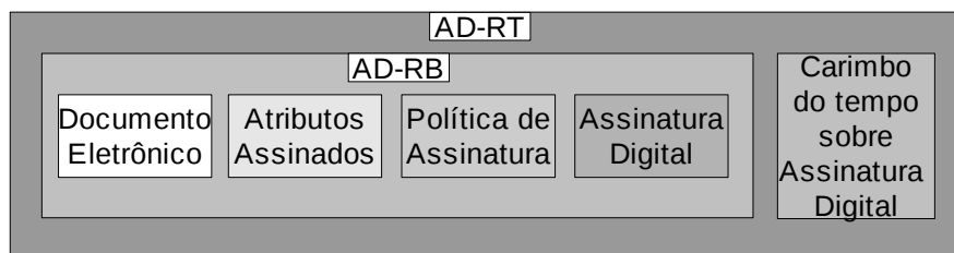
Figura 2.2: Assinatura digital com Referência de Tempo
