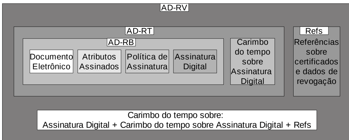
Figura 2.3: Assinatura digital com Referências para Validação
