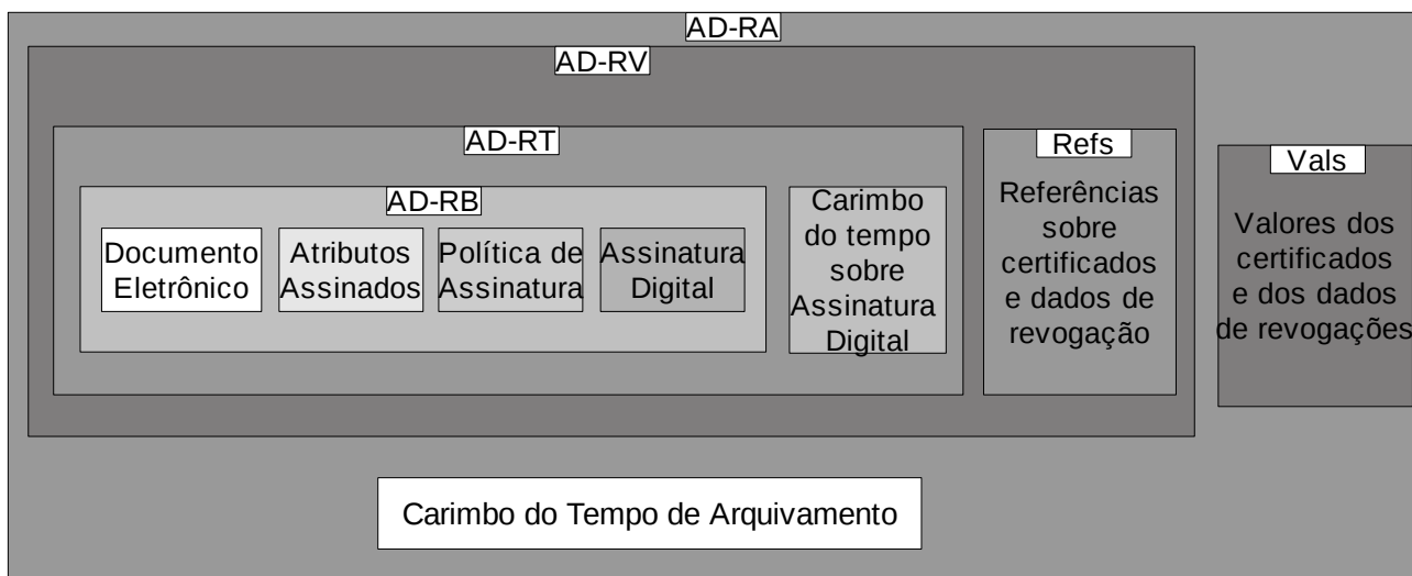
Figura 2.5: Assinatura digital com Referências para Arquivamento
