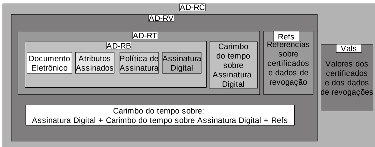
Figura 2.4: Assinatura digital com Referências Completas
