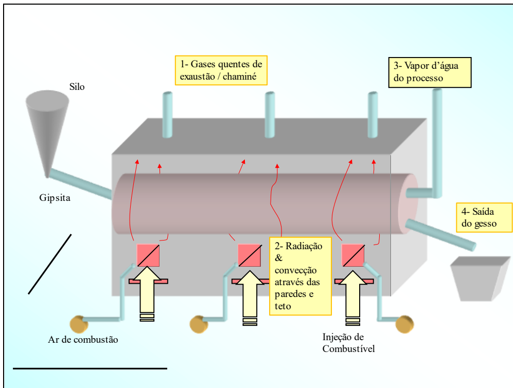
Figura 1 - Representação de um forno calcinador de gipsita e suas perdas de calor (indicadas nas caixas amarelas).
