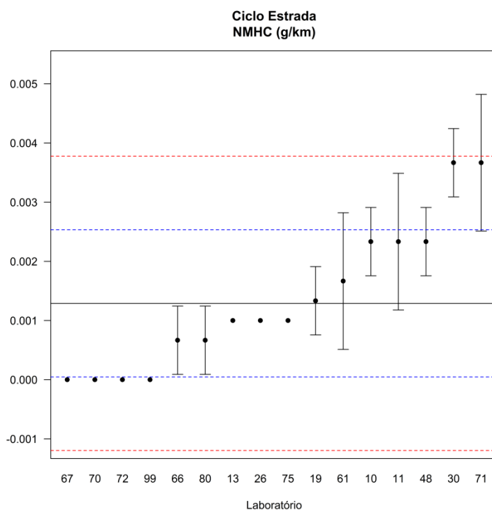
Figura 21 – Gráfico de dispersão dos resultados dos participantes para NMHC – Ciclo Estrada
