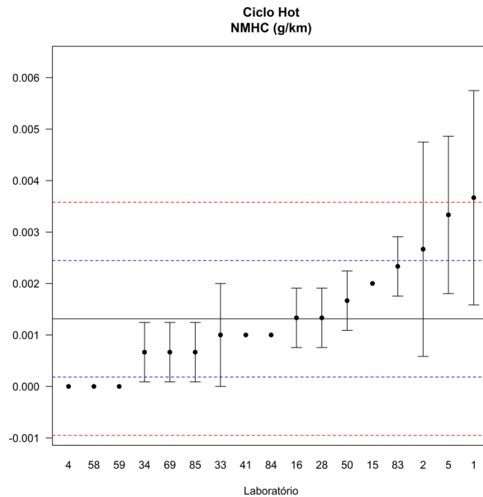
Figura 16 – Gráfico de dispersão dos resultados dos participantes para NMHC – Ciclo HOT
