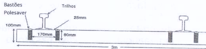
Fig1. Aplicação de Polesaver Rods em dormentes
