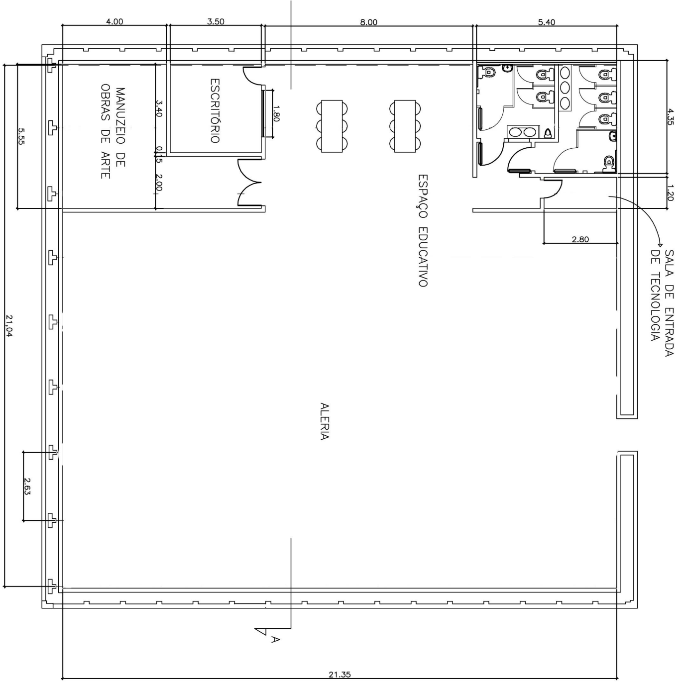
1 PLANTA BAIXA esc.: 1/125
