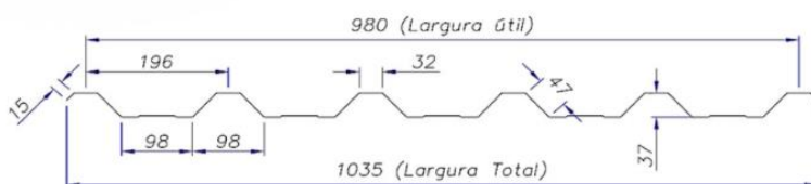
Figura 13 – imagem telha metálica trapezoidal TP40-980
