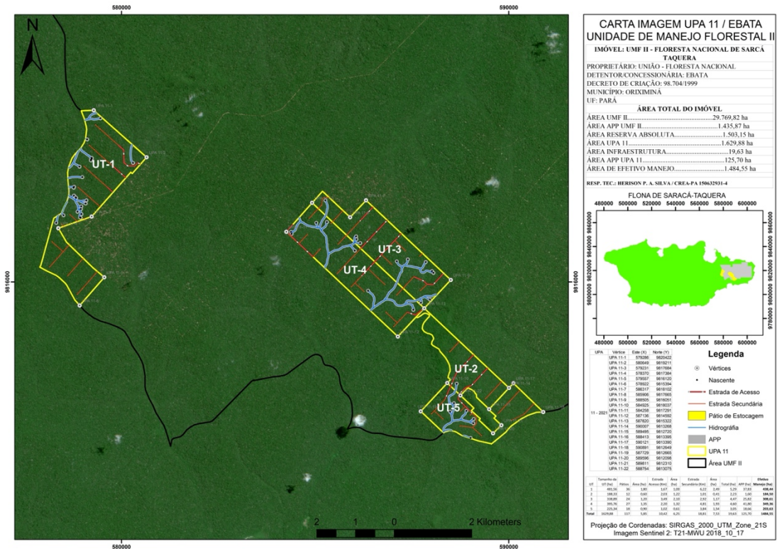
Figura 2: Localização da UPA 11/2022, UMF II, Floresta Nacional Saracá-Taquera, Oriximiná, Pará.
