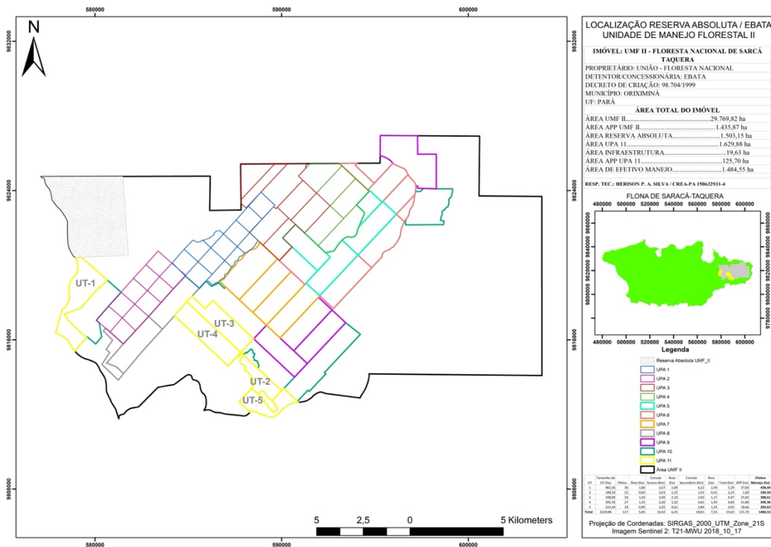
Figura 4: Localização da UPA 11/2022 em relação a área de Reserva Absoluta, Floresta Nacional Saracá-Taquera, Oriximiná, Pará.
