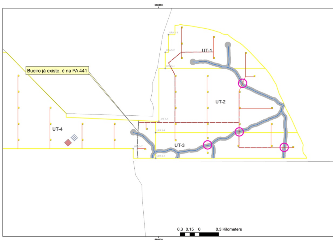
Figura 6: Infraestrutura de bueiros a ser implantada na UPA 3/2017, UMF 1A, Floresta Nacional Saracá-Taquera (Lote-Sul), Terra Santa, Pará.
