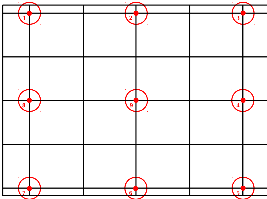
Figura 6: Quantidade e Distribuição de Pontos de Controle (Polinômio do 1º grau - Afim)
