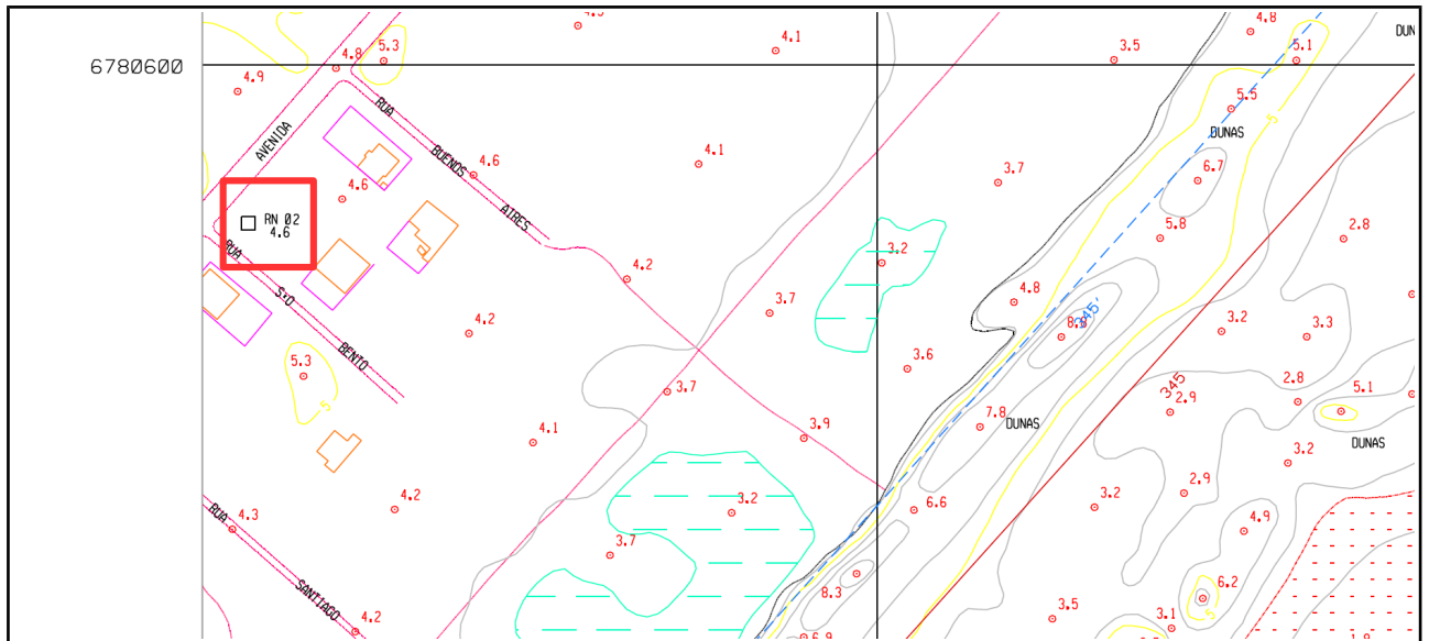
Figura 80: Ponto de Controle (Referência de Nível)
