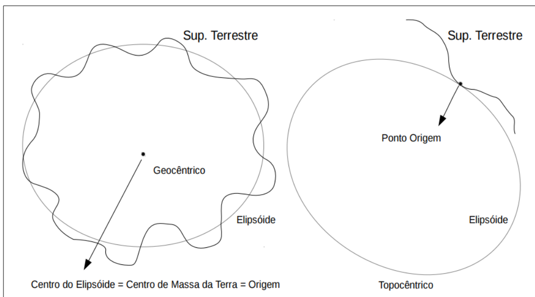
Figura 32: Origem de um Datum Geodésico Planimétrico
