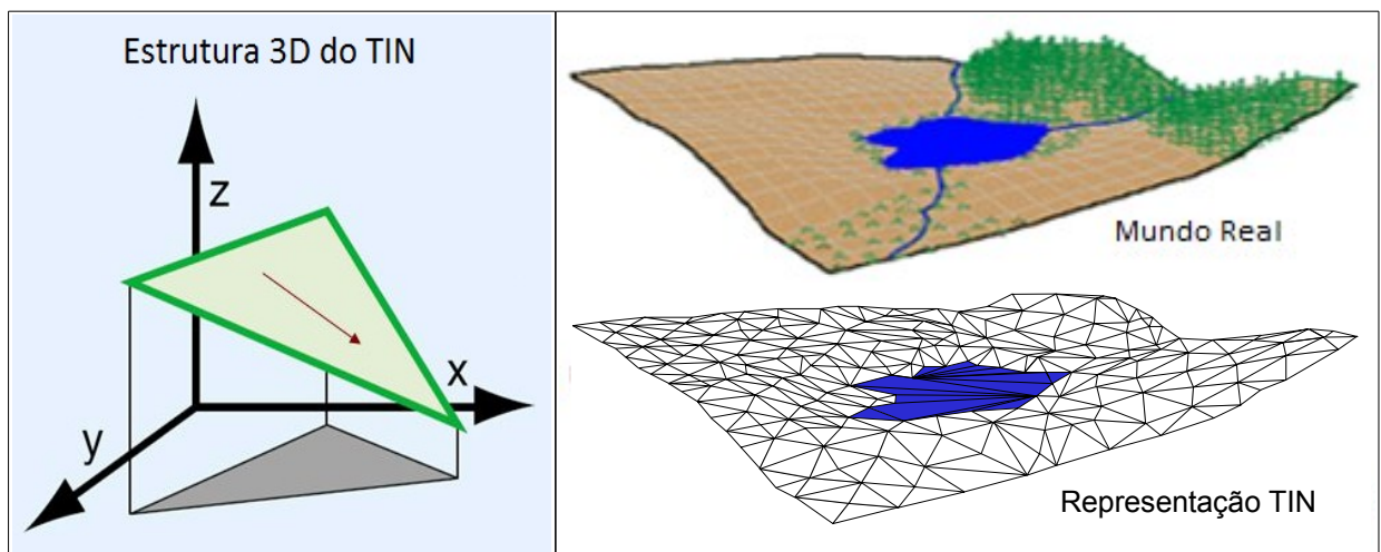
Figura 42: TIN
