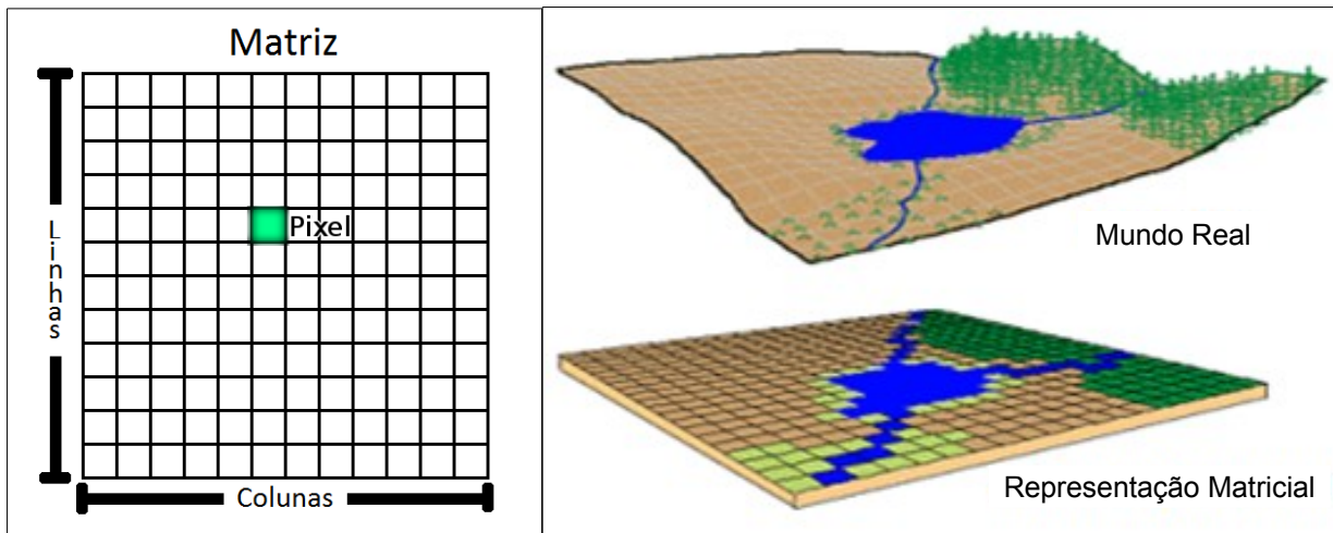
Figura 39: Representação Matricial
