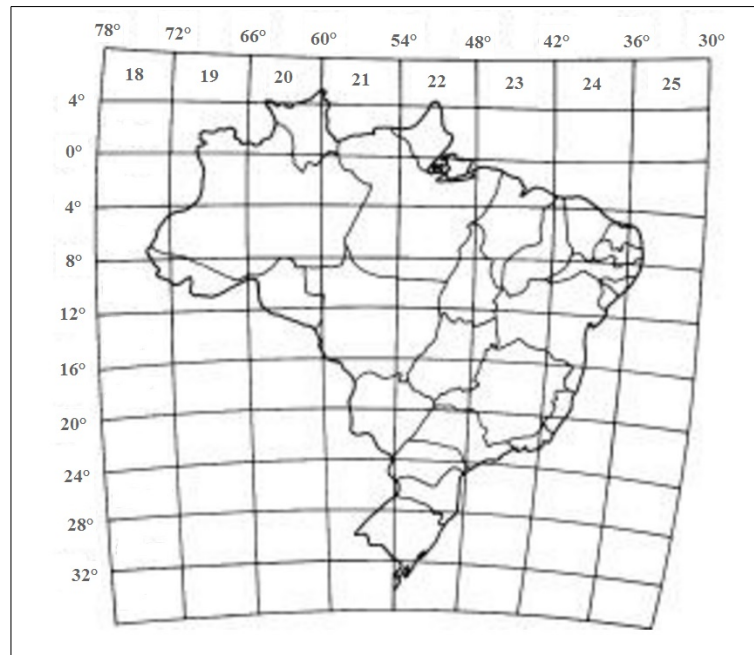
Figura 35: Fusos da Projeção UTM (Brasil)
