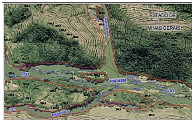
Figura 15: Ortofotocarta
