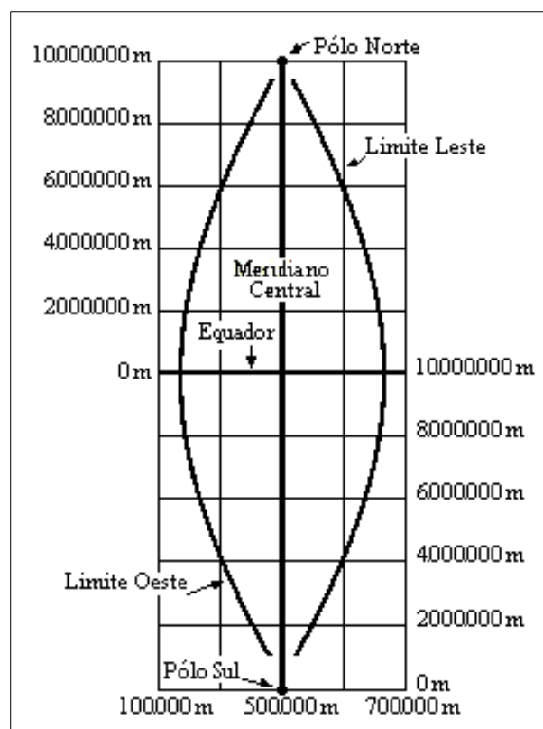
Figura 36: Coordenadas E e N da Projeção UTM (Fuso)
