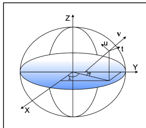
Figura 28: Sistema Geodésico Local, onde o eixo u (N) aponta em direção ao norte geodésico, o eixo t (E) aponta para Leste e é perpendicular ao eixo u; ambos estão contidos no plano topográfico. O eixo v (U) coincide com a normal ao elipsóide que passa pelo ponto considerado, que determina a origem do sistema.
