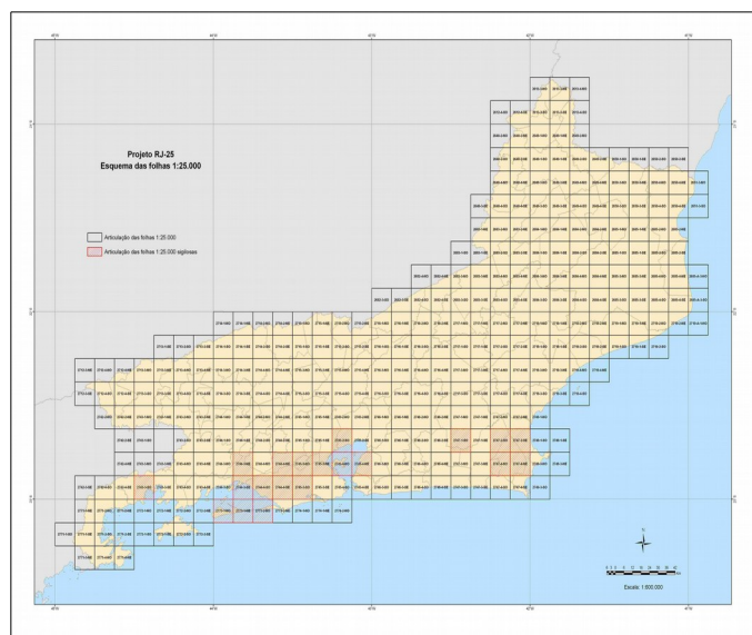
Figura 8: Carta Índice
