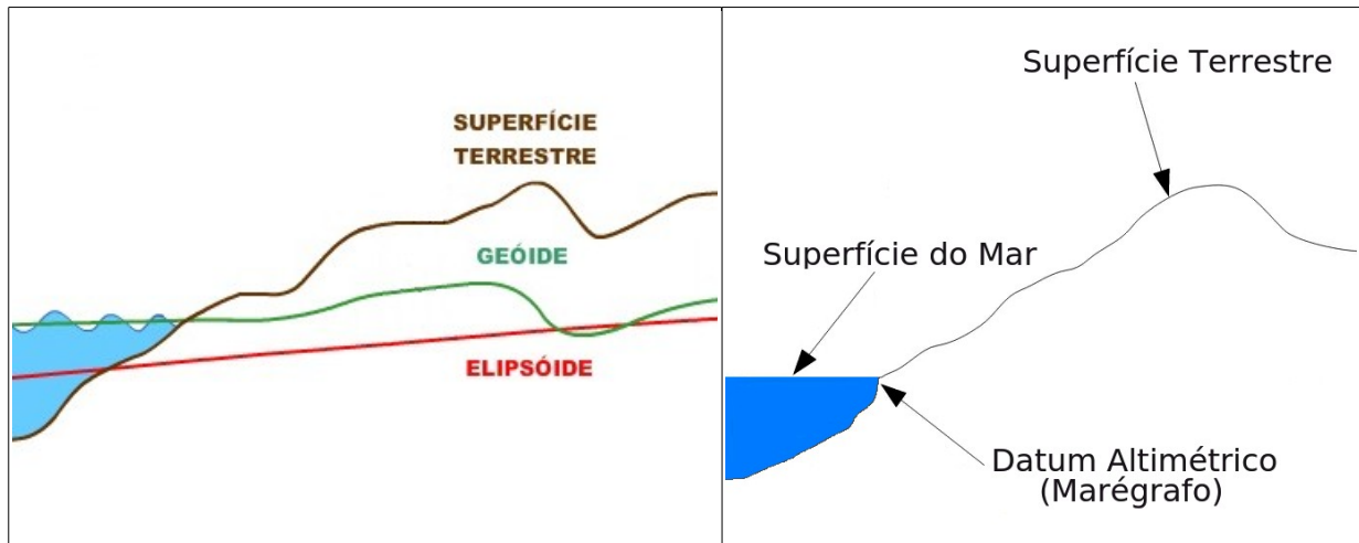
Figura 56: Geóide e Datum Geodésico Altimétrico
