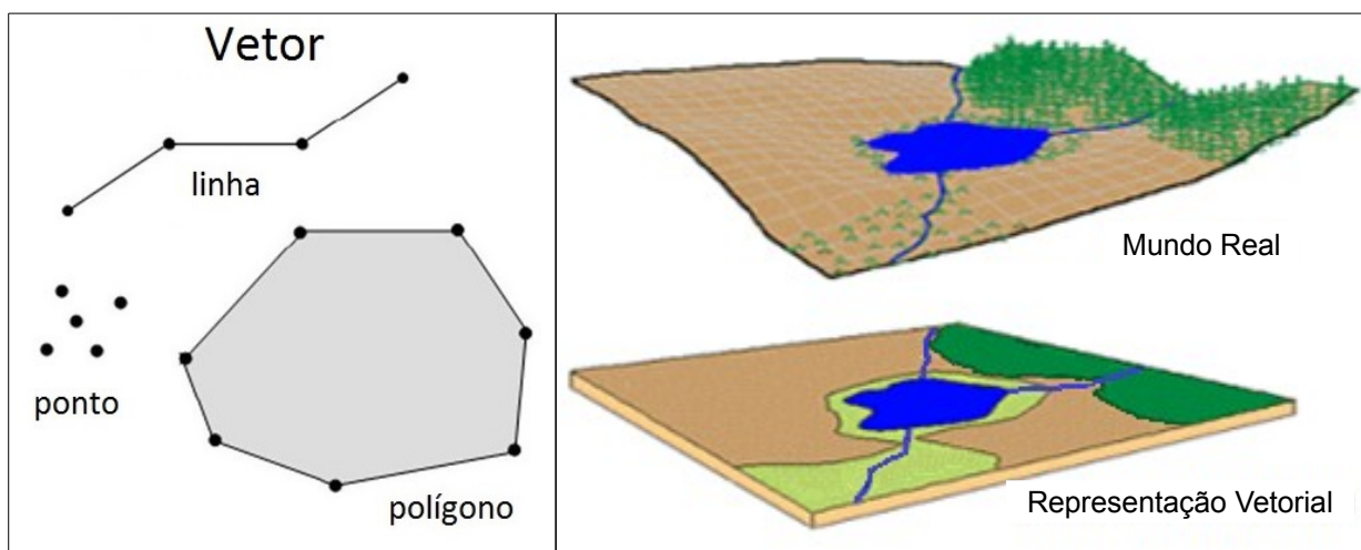
Figura 40: Representação Vetorial
