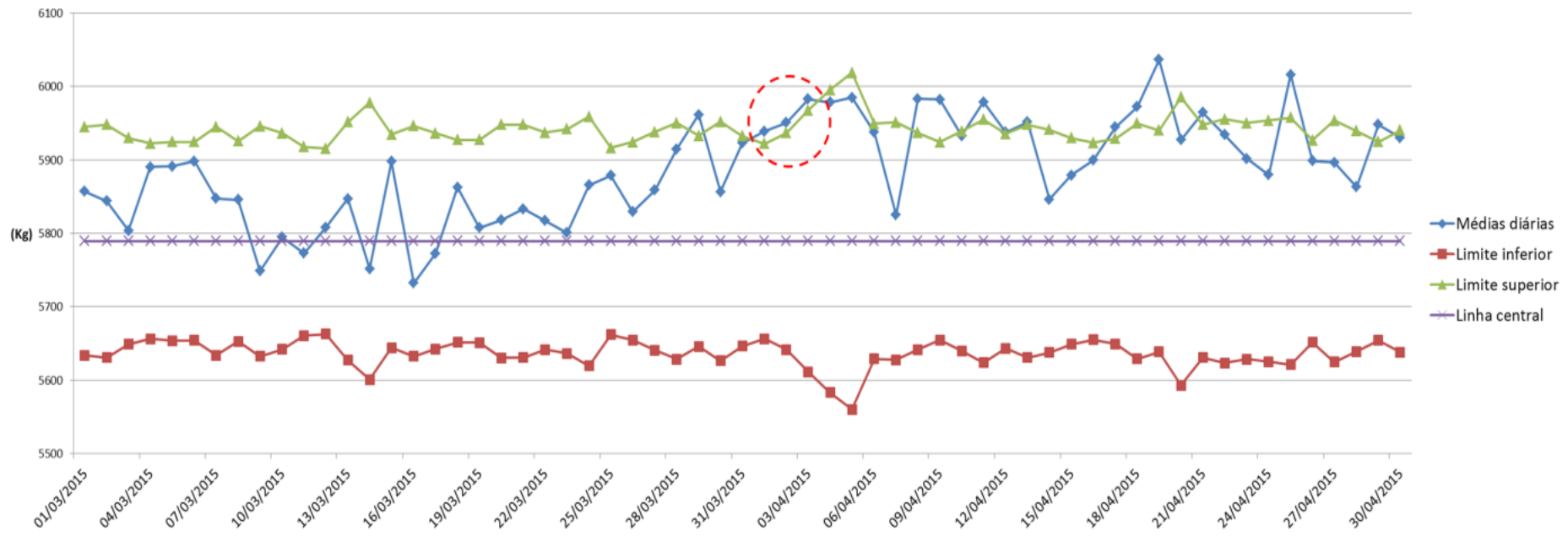
Xbar peso 1º eixo E1/3S3 - Estação Integrada - Março e Abril 2015
