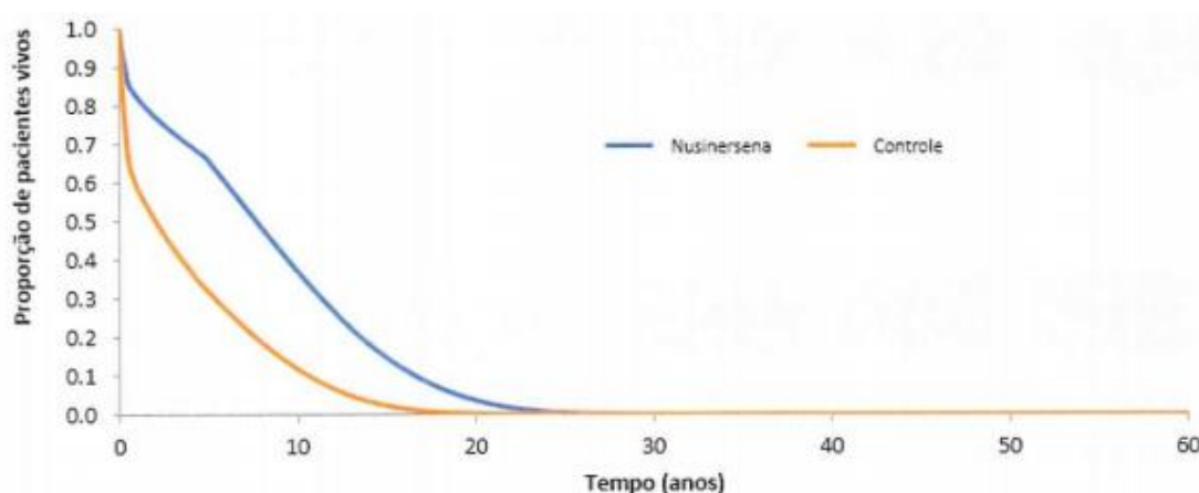
Figura 7: Curvas de sobrevida utilizadas no modelo de AME 5q início precoce
