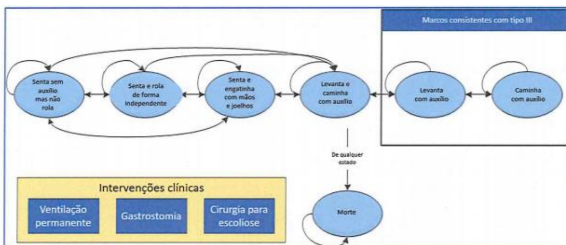
Figura 12: Estrutura do modelo de Markov para AME 5q início tardio
