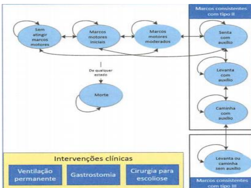
Figura 8: Estrutura do modelo de Markov proposto
