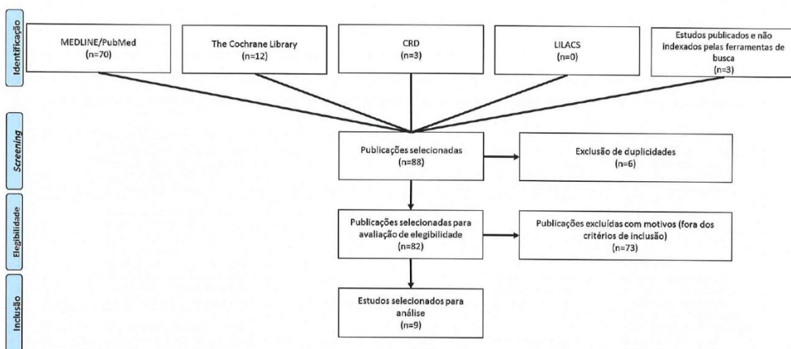
Figura 7. Fluxograma de seleção de estudos.
