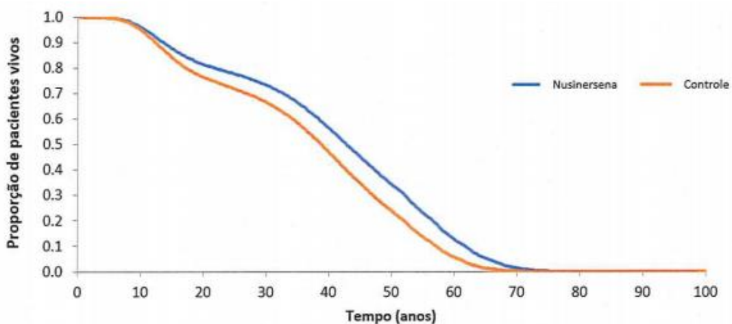
Figura 13: Curvas de sobrevida utilizadas no modelo AME 5q início tardio
