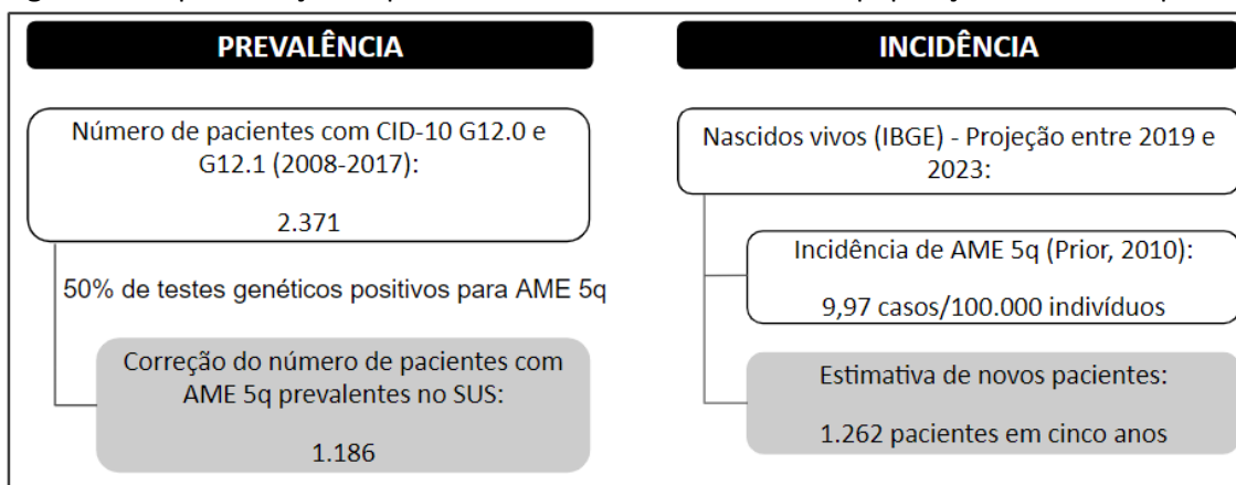
Figura 16: Representação esquemática do método de cálculo da população com AME 5q
