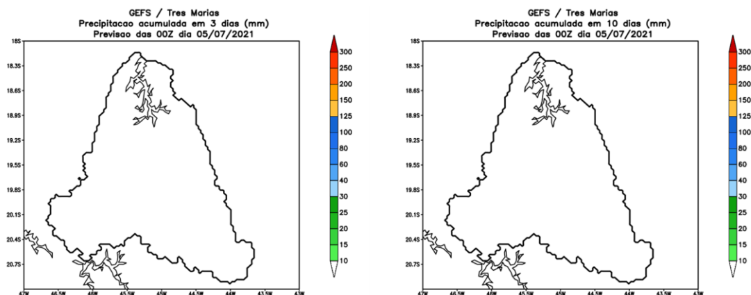
Figura 4. Previsão de precipitação acumulada em milímetros (mm) nos próximos 3 (esquerda) e 10 (direita) dias para a bacia de captação do Aproveitamento Hidrelétrico Três Marias, segundo a previsão do modelo numérico GENS/NOAA. A área da bacia de captação do aproveitamento hidrelétrico de Três Marias é indicada na Figura com linha preta espessa.
