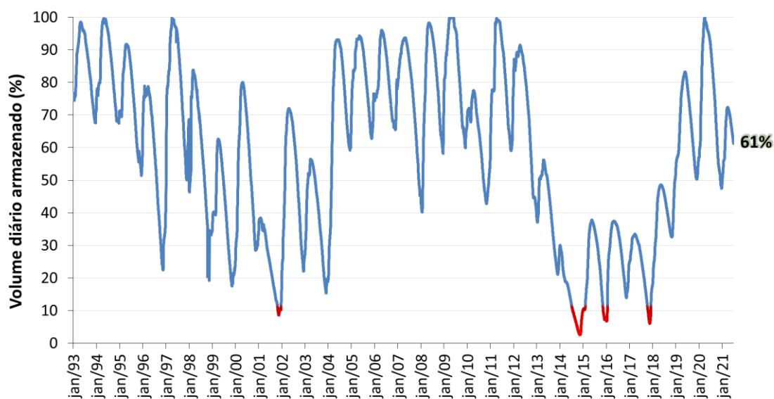
Figura 3. Evolução do volume diário armazenado do Aproveitamento Hidrelétrico Três Marias até 30 de junho de 2021 (em porcentagem). Fonte dos dados: Sistema de Acompanhamento de Reservatórios/ANA.
