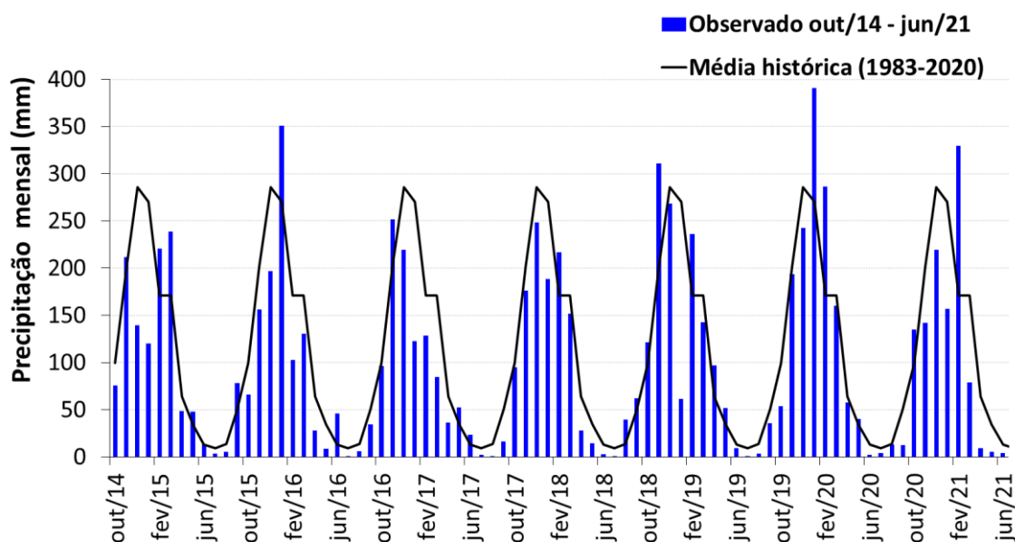
Figura 1. Precipitação mensal na bacia hidrográfica afluente ao Aproveitamento hidrelétrico Três Marias (ano hidrológico: outubro-setembro).
