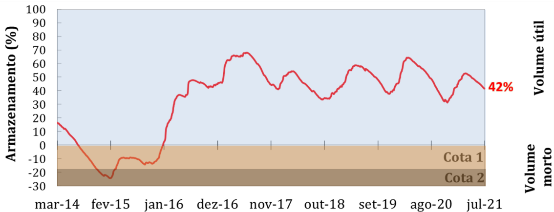
Figura 6. Evolução diária do nível de armazenamento (%) do Sistema Cantareira. Área em azul corresponde ao volume útil do reservatório (982 hm 3 ), em marrom claro à primeira cota do volume morto (182,5 hm 3 ) e em marrom escuro à segunda cota do volume morto (105 hm 3 ). Fonte dos dados: SABESP.
