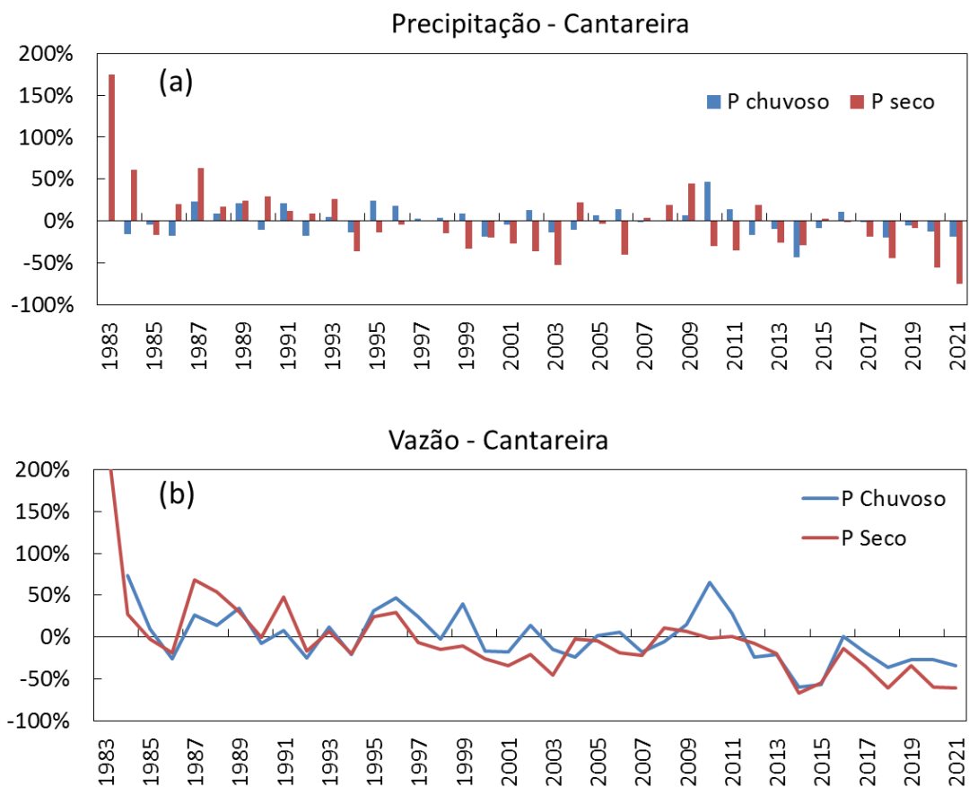
Figura 2. Anomalia de (a) precipitação (P) e (b) vazão (Q) sazonais para o Sistema Cantareira. Período seco: abril a setembro. Período chuvoso: outubro a março.
